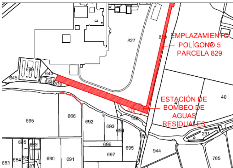
Estación de bombeo de aguas residuales fuera de los límites de la Vía Pecuaria
