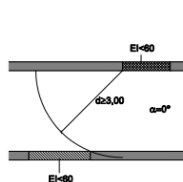
Figura 1.1. Fachadas enfrentadas
