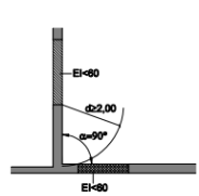
Figura 1.4. Fachadas a 90°
