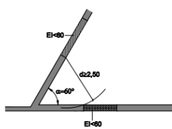
Figura 1.3. Fachadas a 60°
