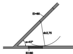
Figura 1.2. Fachadas a 45°
