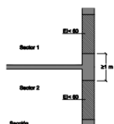
Figura 1.7 Encuentro forjado-fachada
