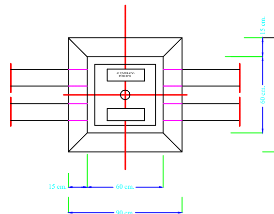
PLANTA DE ARQUETA DE CRUCE
