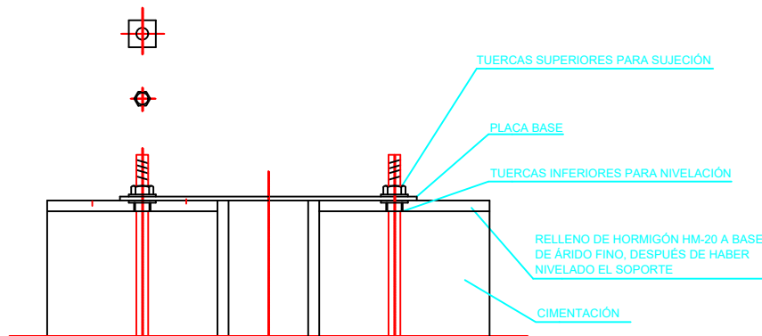
DETALLE SISTEMA DE NIVELACIÓN ESCALA 1:5
