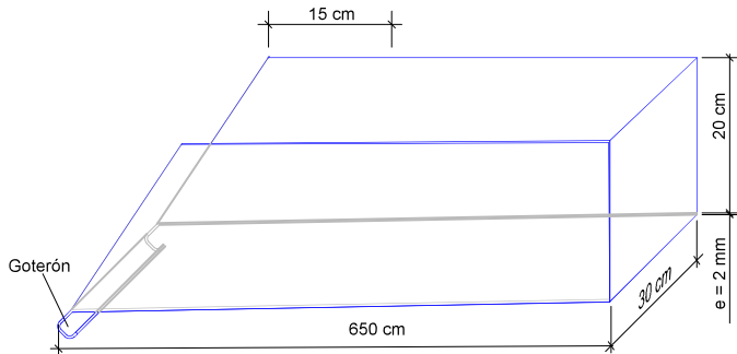
DETALLE 3D ALBAÑAL INOXIDABLE A3 = 1/10 A1 = 1/5
