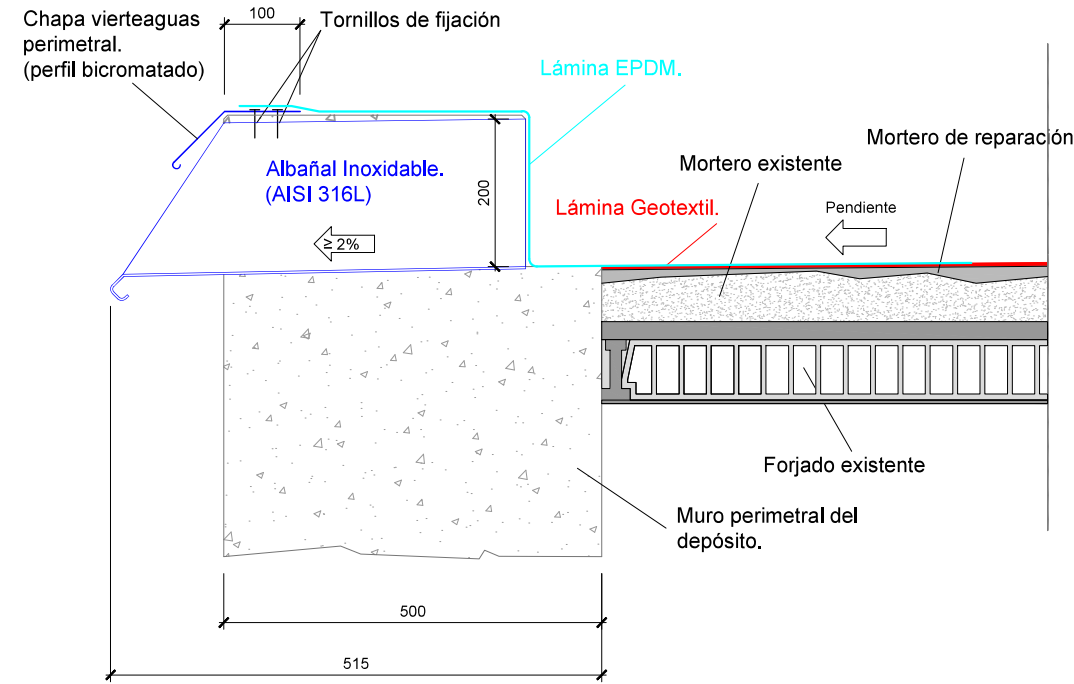
SECCIÓN EN ALZADO DE ALBAÑAL Y LÁMINA EPDM COLOCADOS A3 = 1/10 A1 = 1/5
