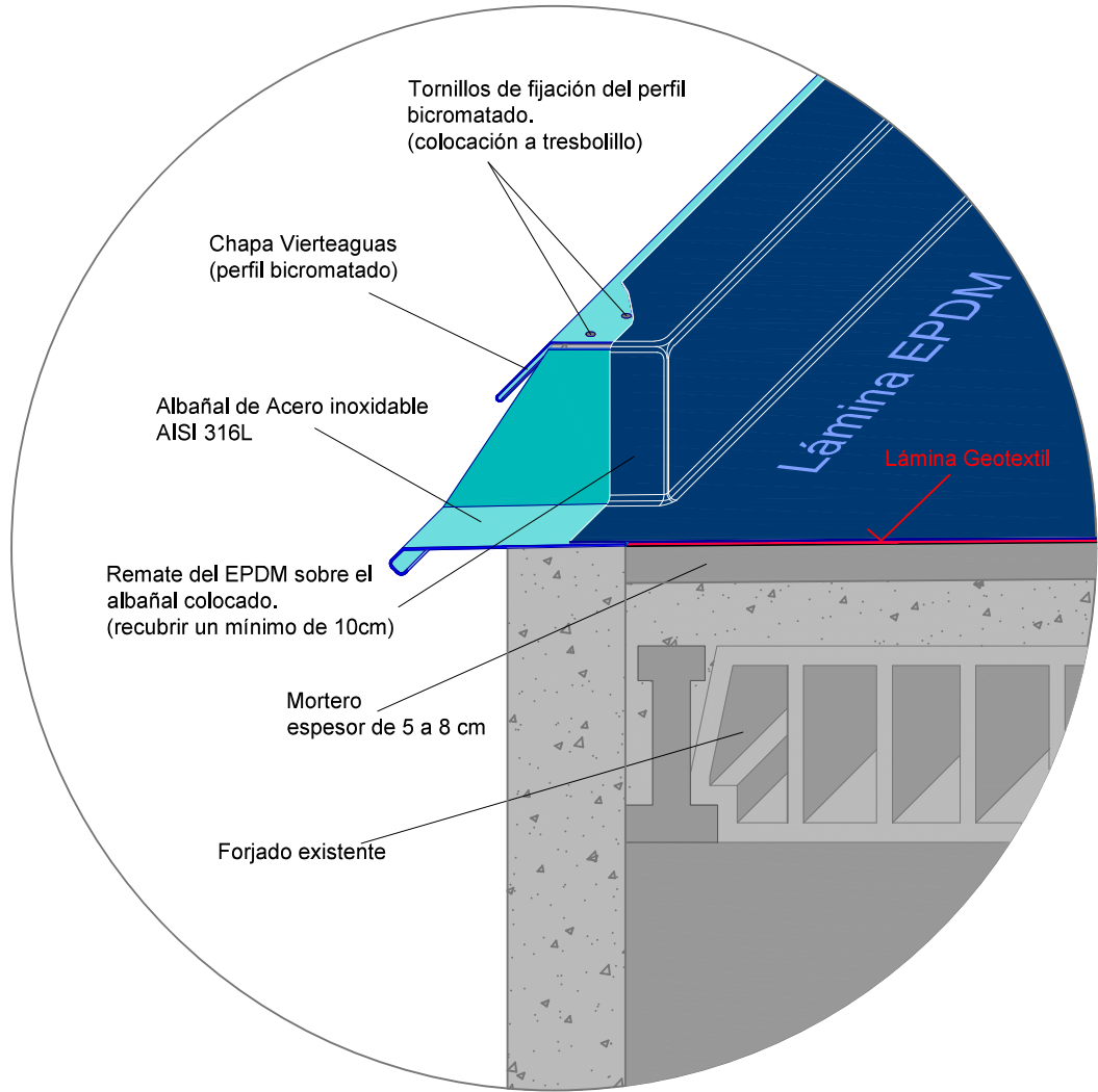
DETALLE 3D ALBAÑAL Y EPDM COLOCADOS A3 = 1/10 A1 = 1/5
