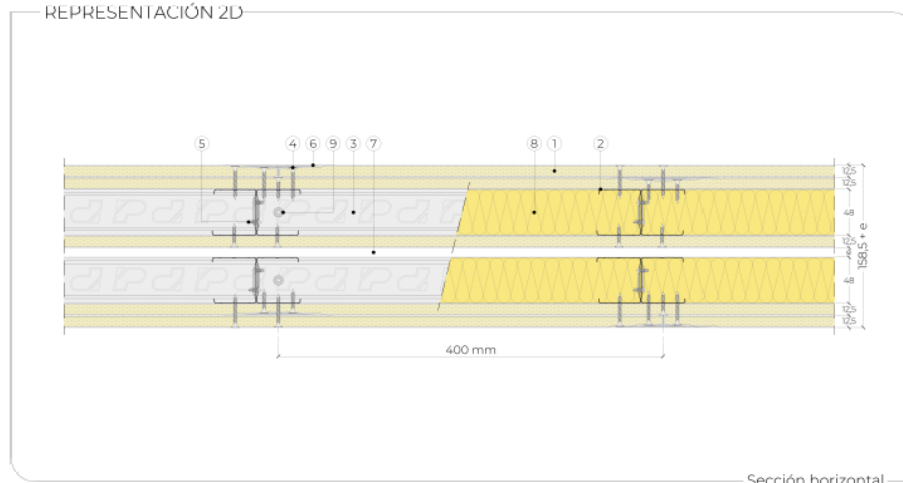
Sección horizontal
