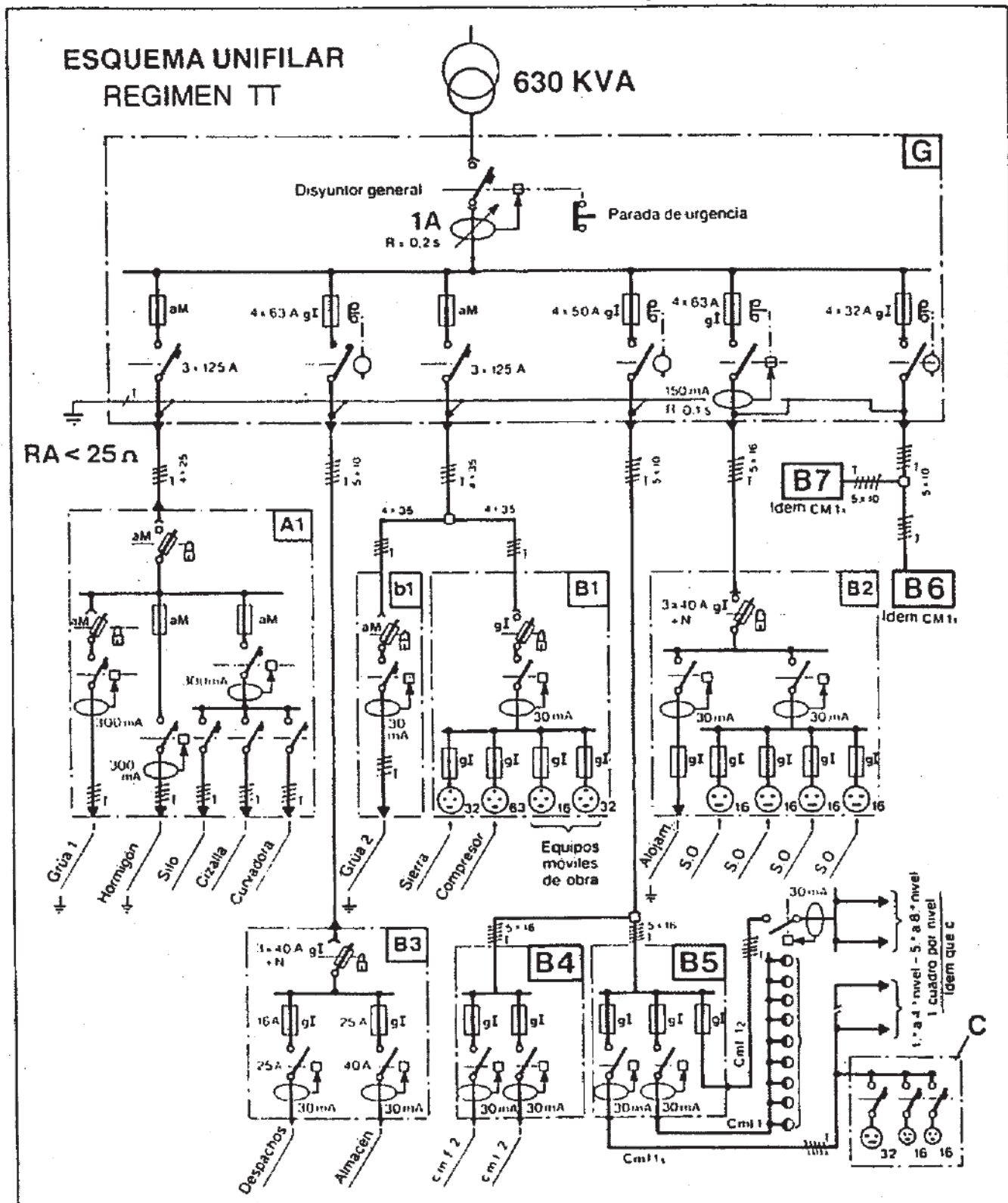
Fig. 45.- Esquema eléctrico de una gran obra.
