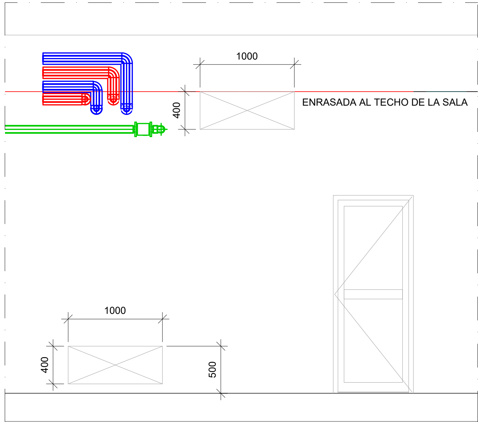
SECCIÓN B-B' - REJILLAS DE VENTILACIÓN
