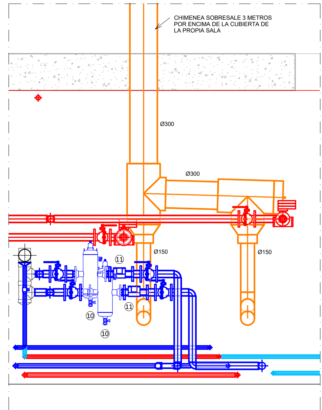
SECCIÓN A-A'
