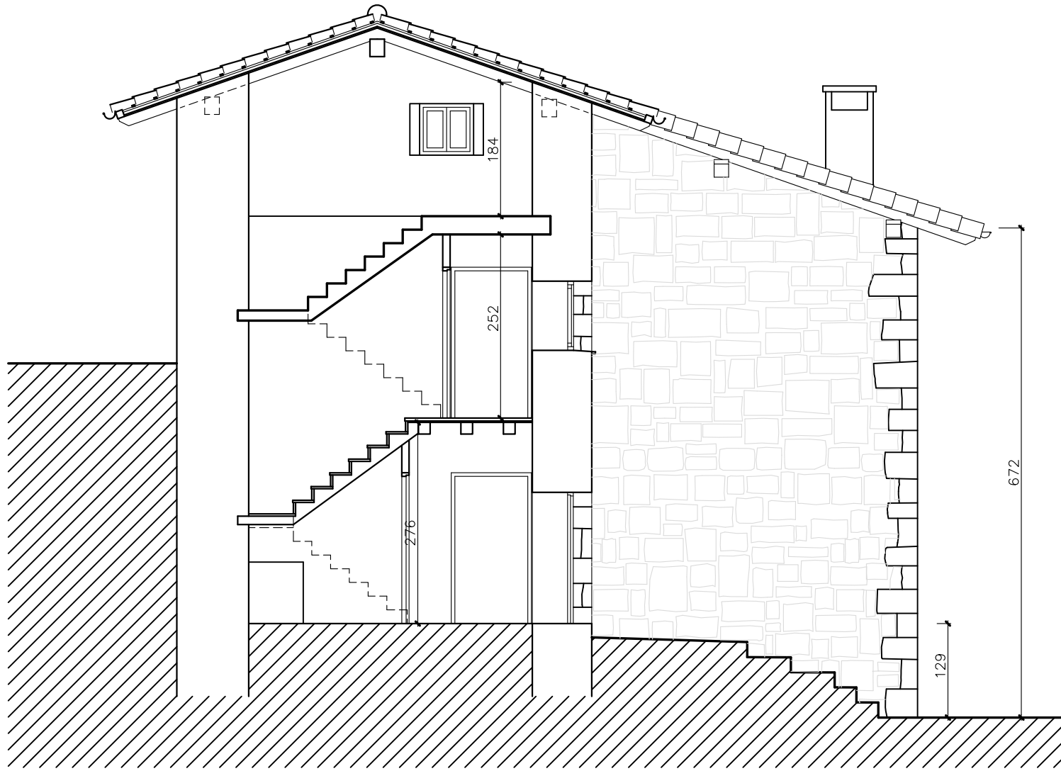
SECCION S.1.
