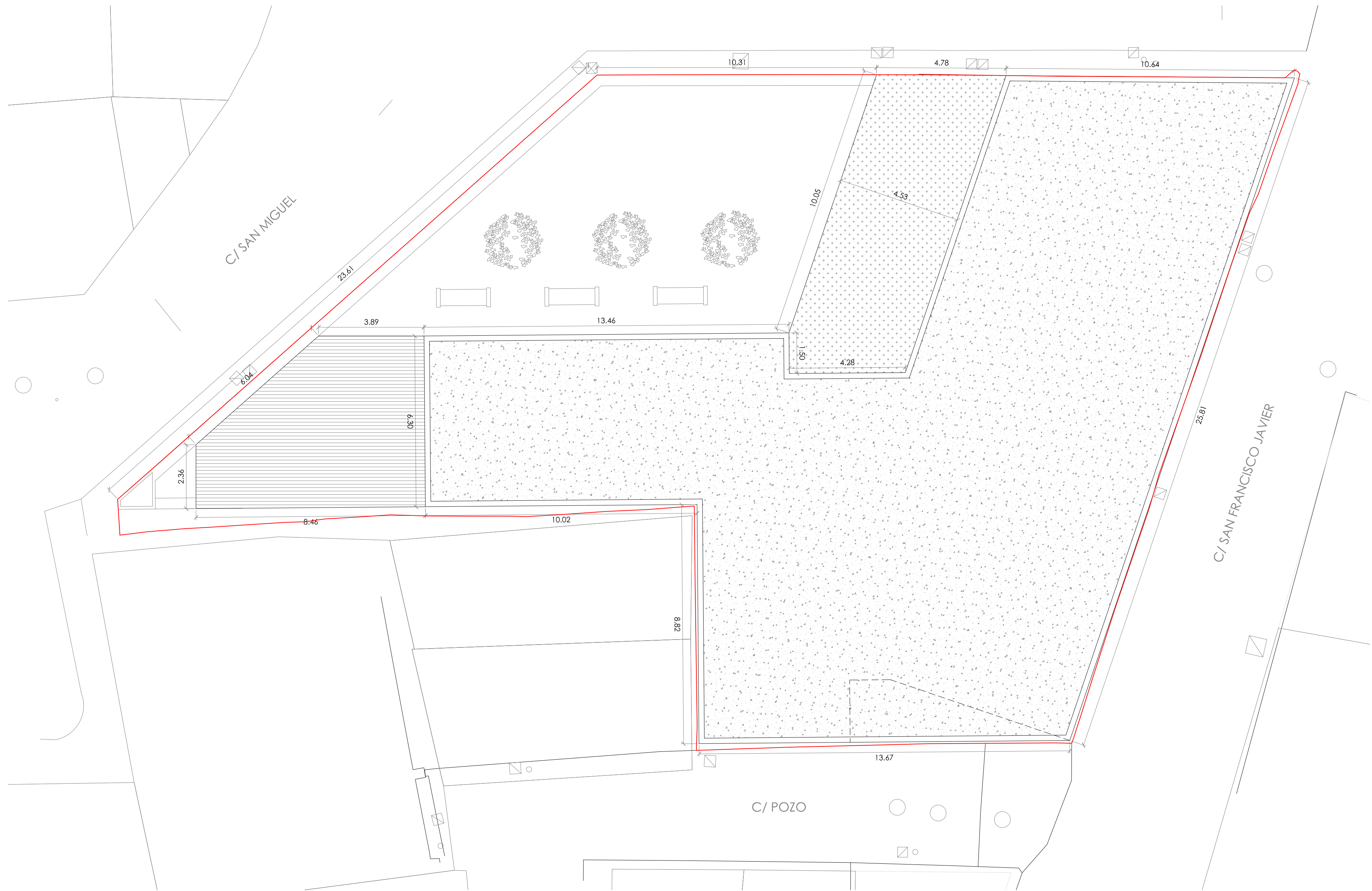
CUBIERTA PROPUESTA
