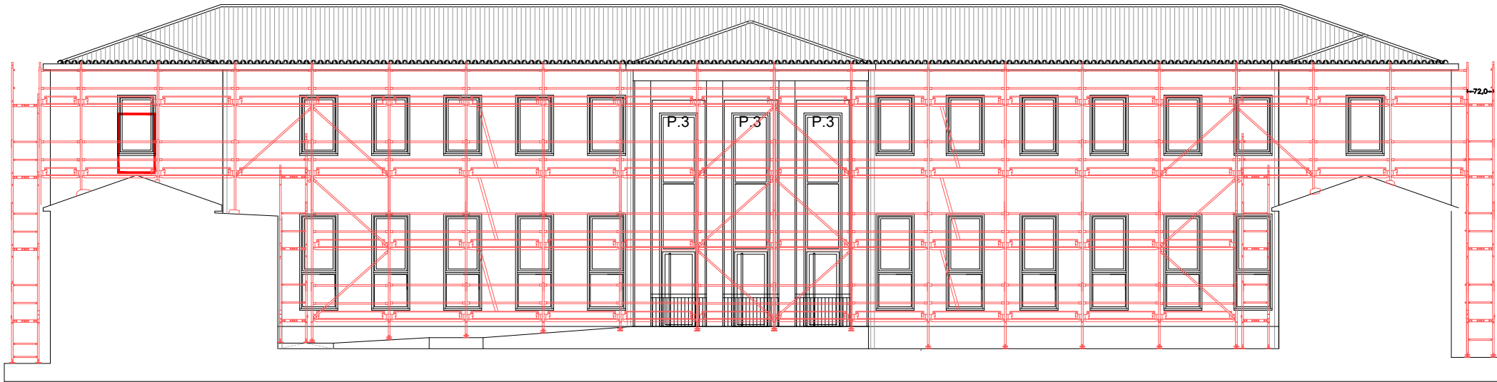
ALZADO FACHADA OESTE _PATIO INTERIOR
