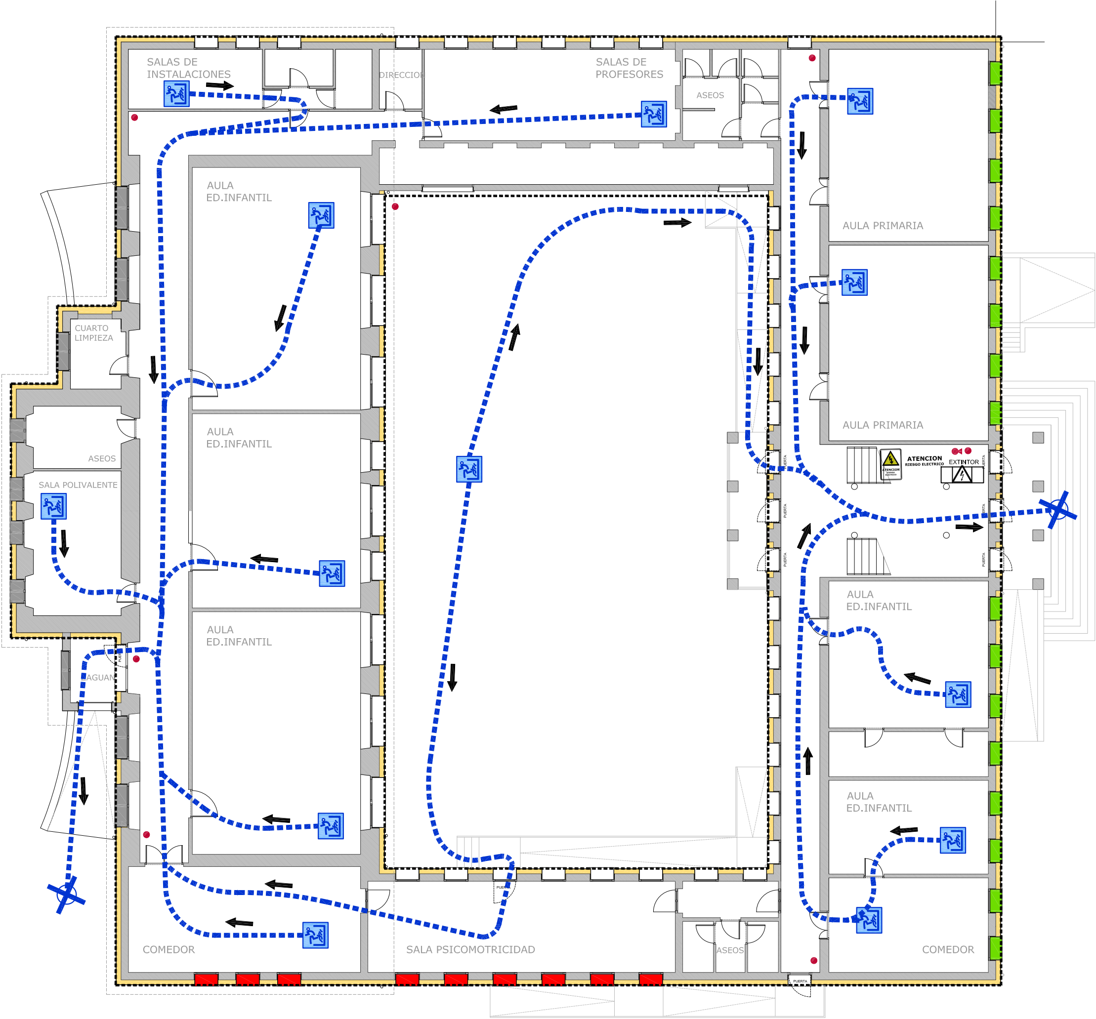
PLANTA BAJA
