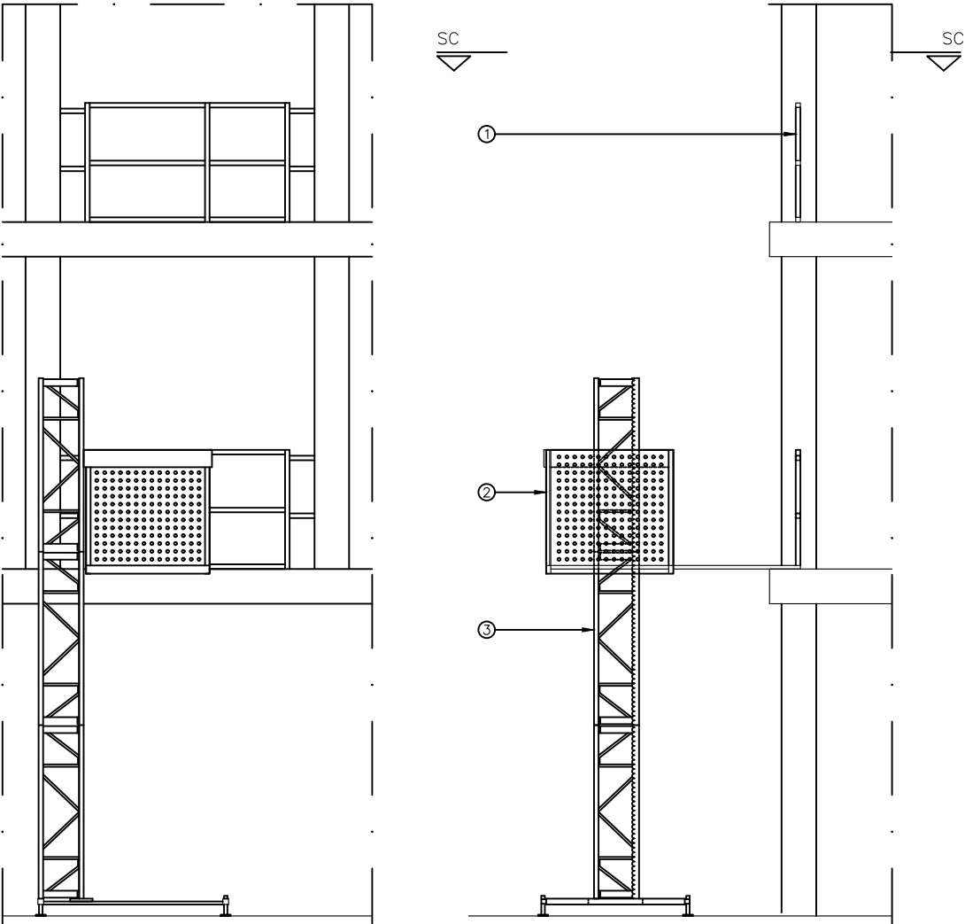
SECCIÓN A-A
