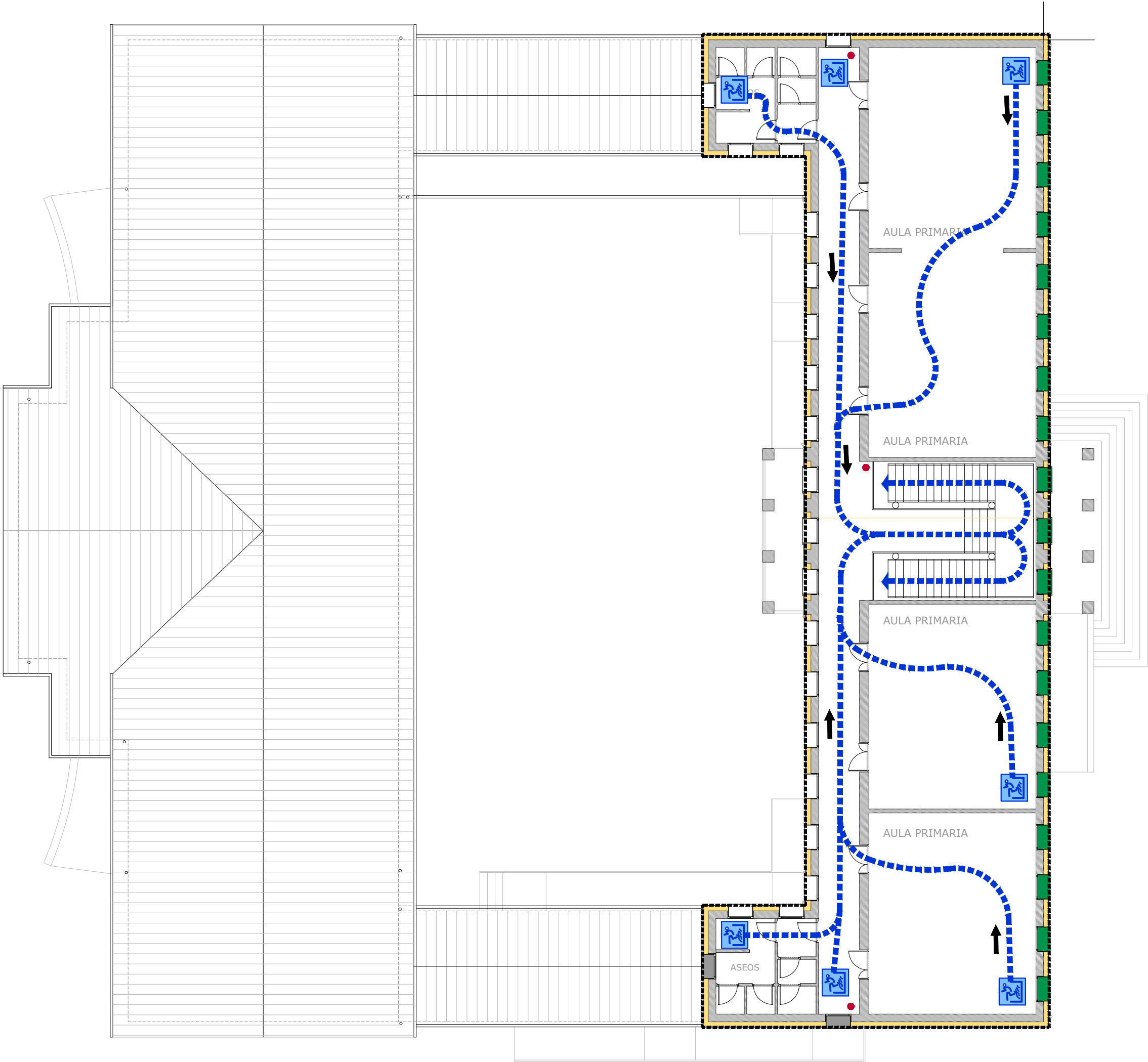
PLANTA PRIMERA
