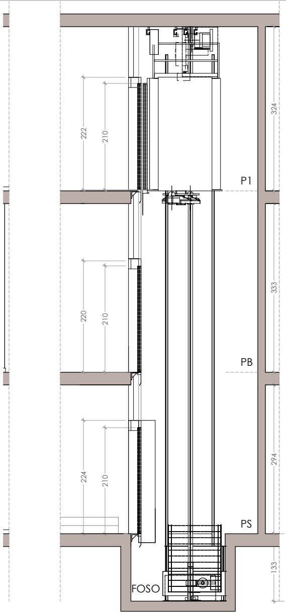
SECCIÓN B-B' - e:1/75
