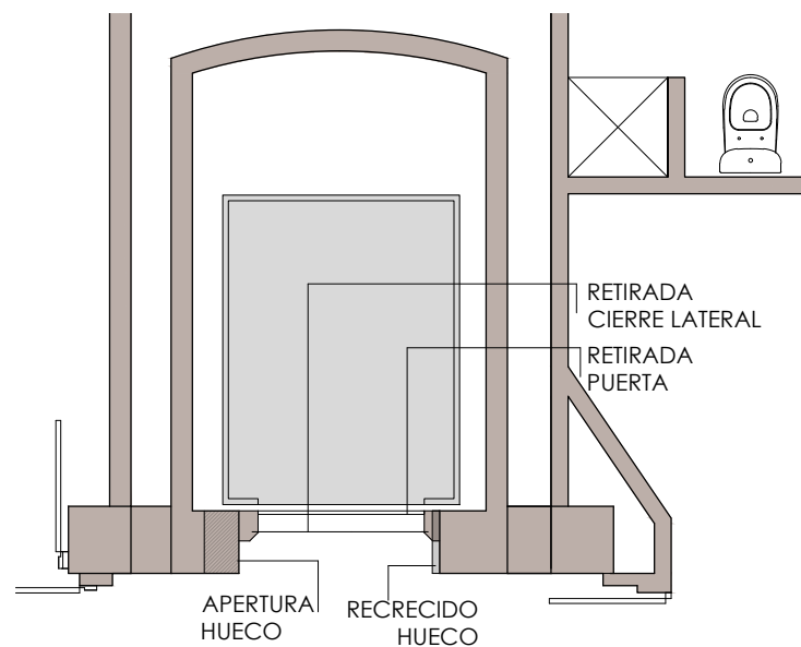
PLANTA PRIMERA
