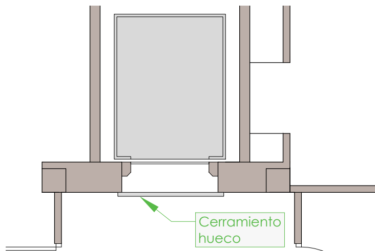
PLANTA SOTANO
