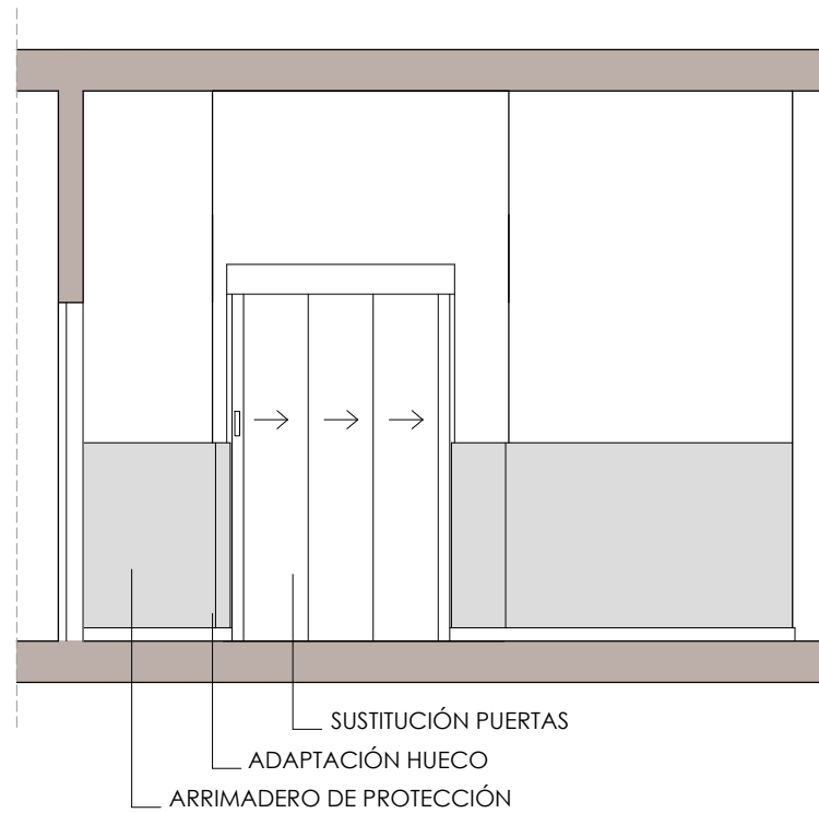
ALZADO PLANTA BAJA
