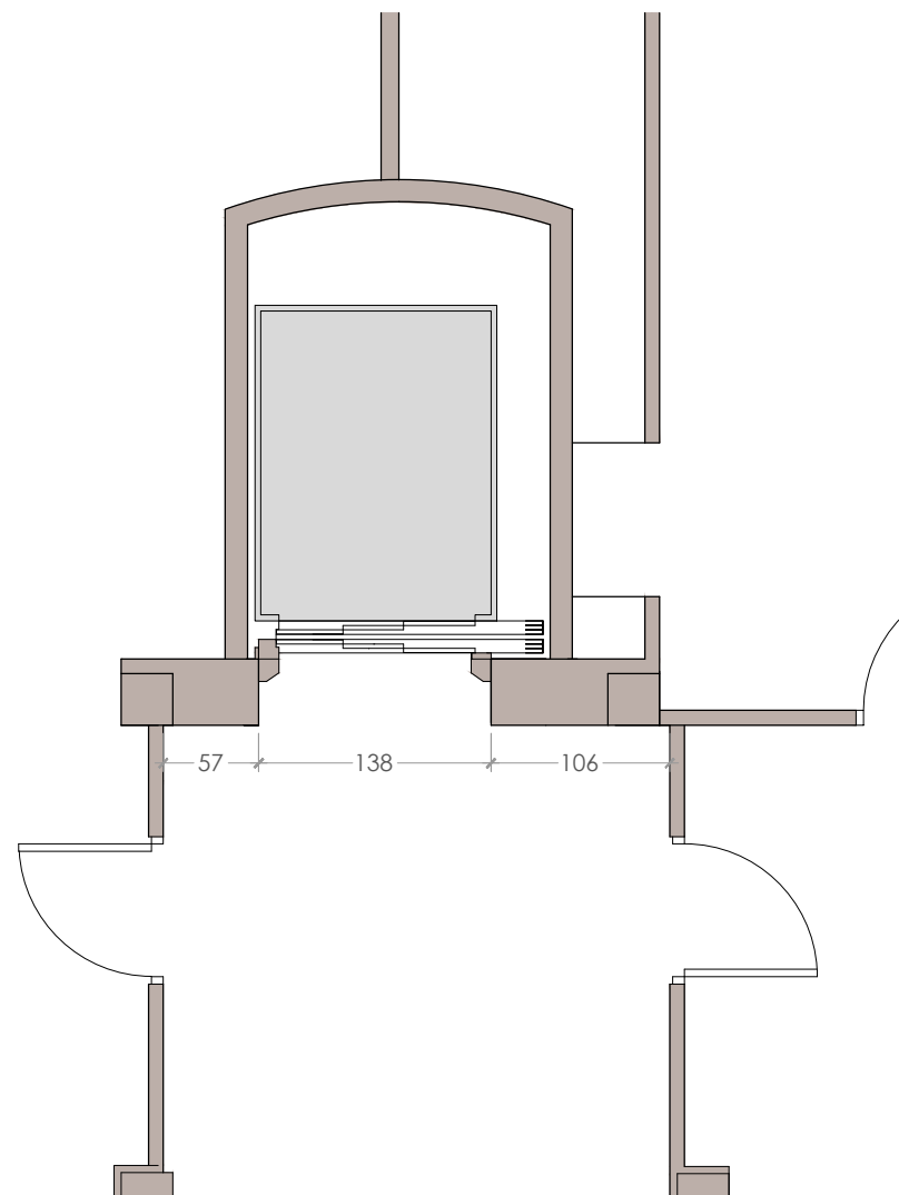
PLANTA SOTANO
