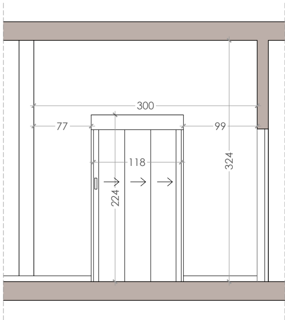
ALZADO PLANTA PRIMERA
