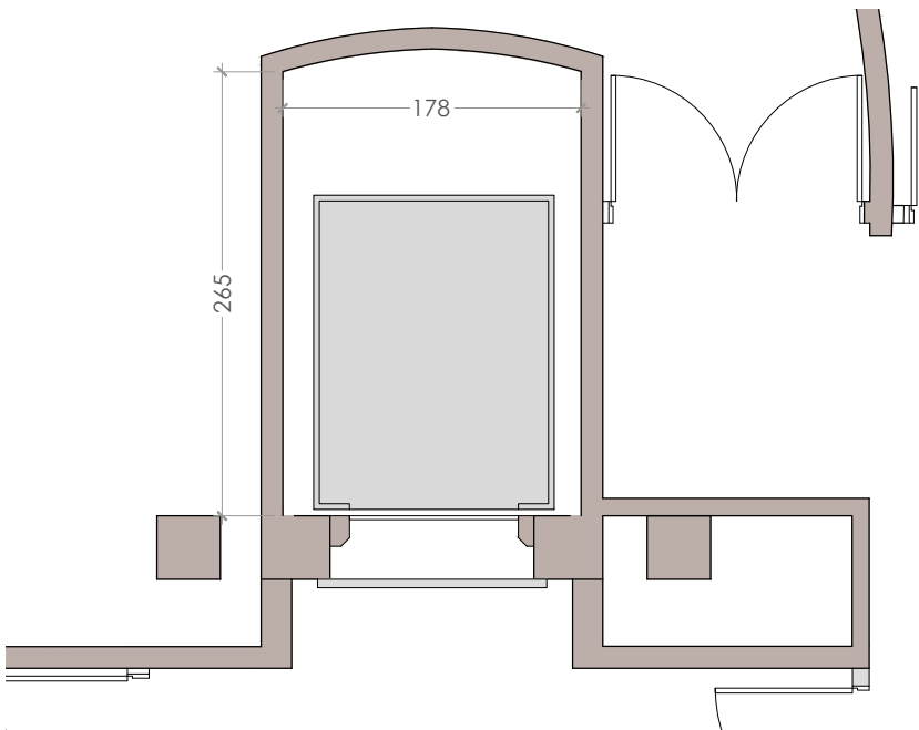
PLANTA BAJA
