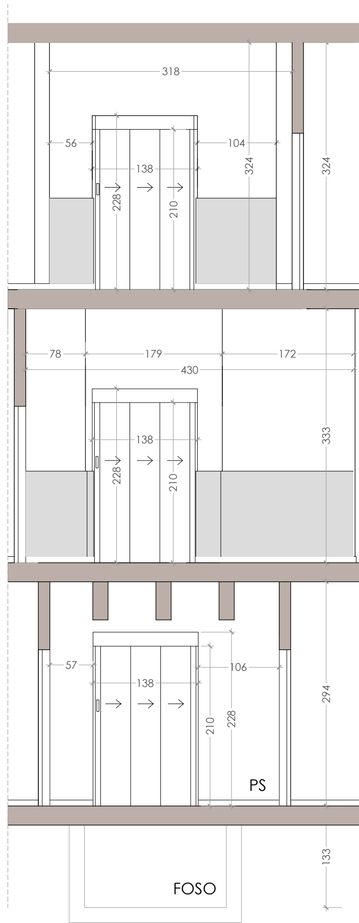
SECCIÓN AÁ
