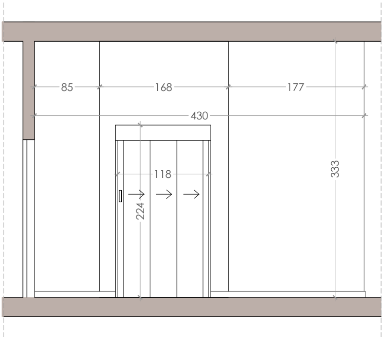
ALZADO PLANTA BAJA
