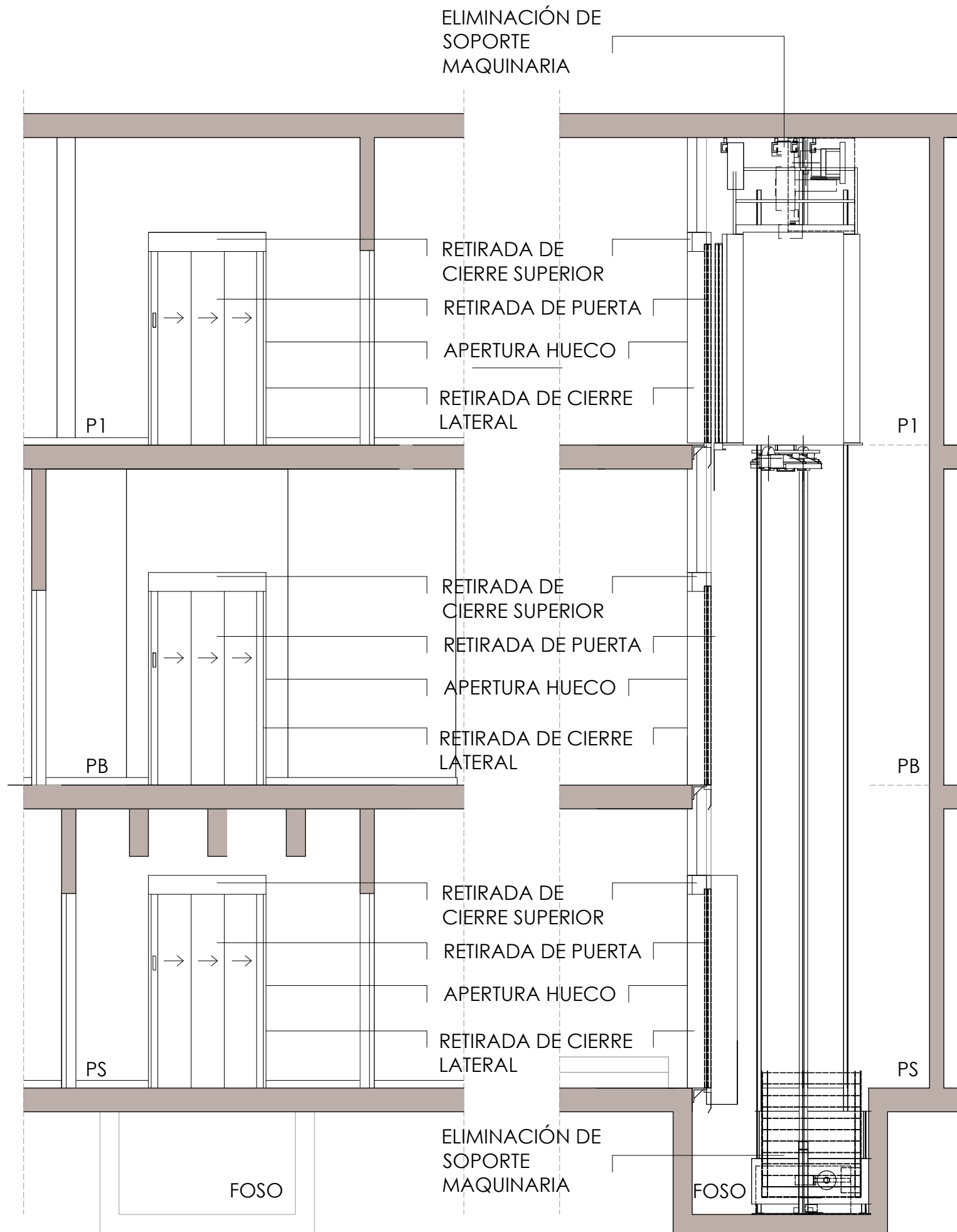
SECCIÓN AA
