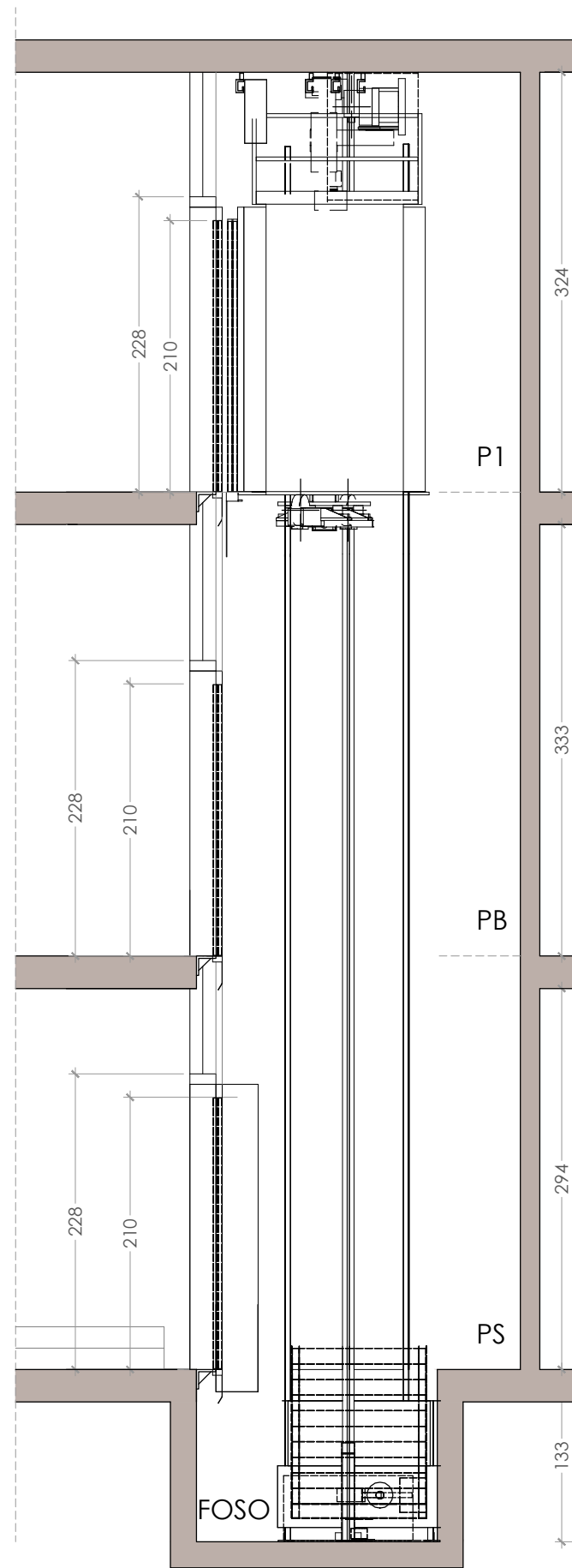
SECCIÓN BB´
