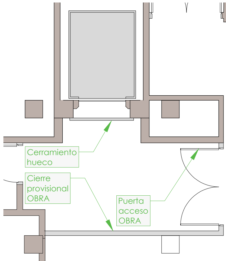
PLANTA BAJA
