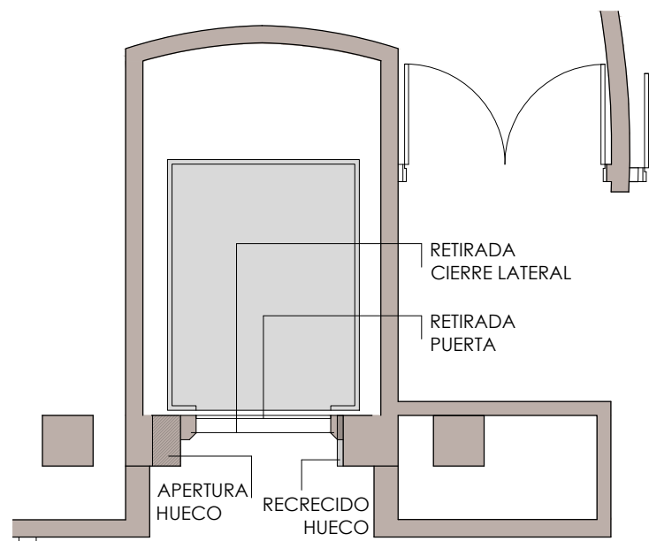
PLANTA BAJA
