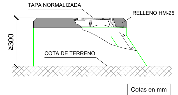
DETALLE DE REMATE EN CAMPO DE TAPA DE REGISTRO E=1/20
