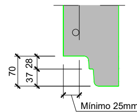
DETALLE - B (cotas en mm)
