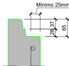
DETALLE - A (cotas en mm)
