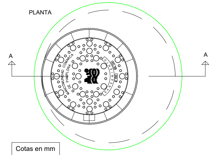
DETALLE DE LA JUNTA ENTRE MÓDULOS E=1/10
