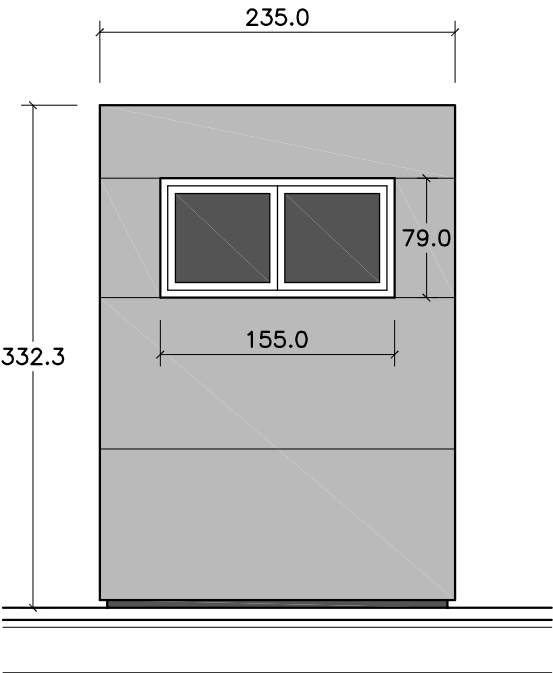
ALZADO NORTE
