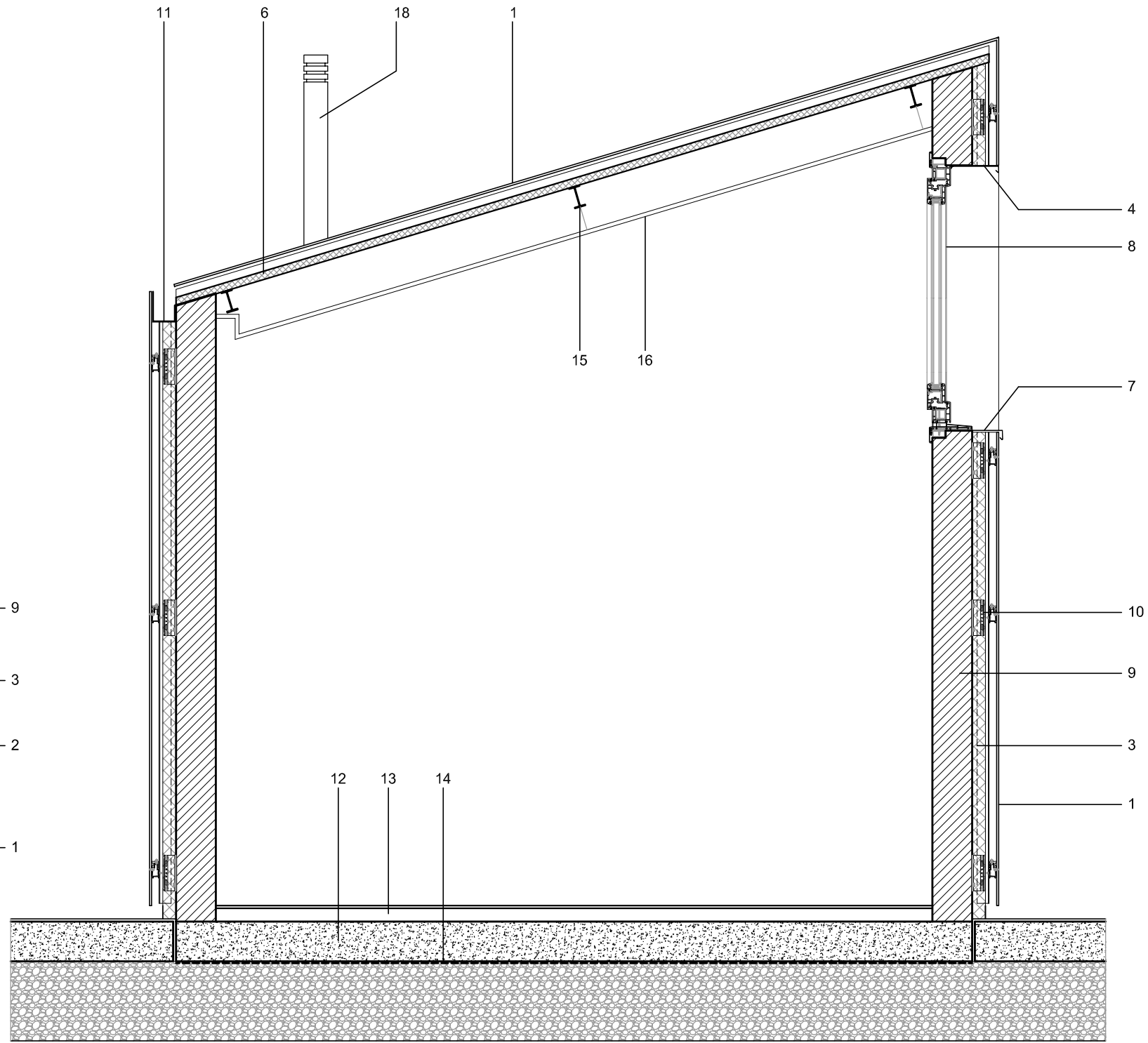
SECCIÓN
