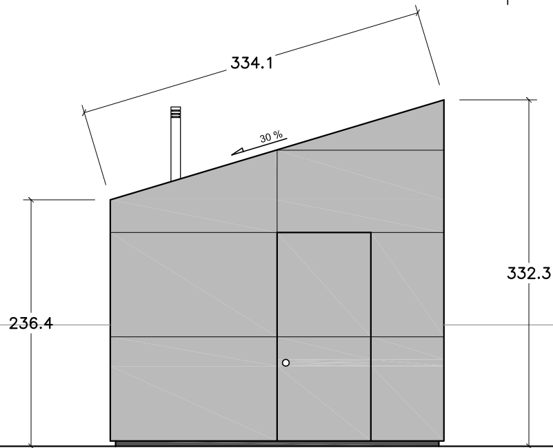
ALZADO ESTE
