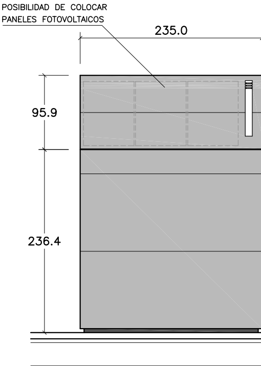
ALZADO SUR
