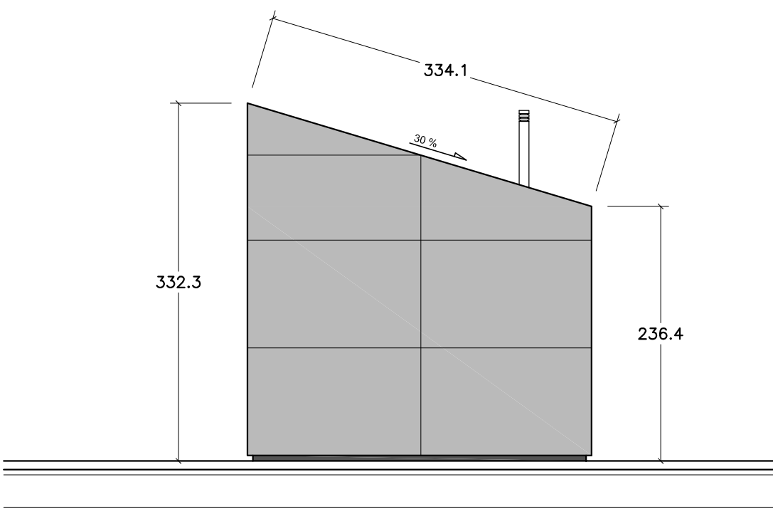
ALZADO OESTE
