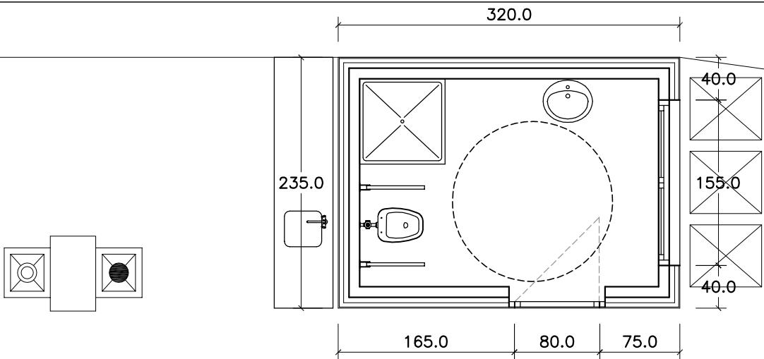
PLANTA
