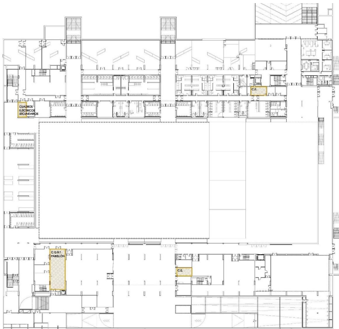
Planta sótano -1. Posición cuartos eléctricos.
