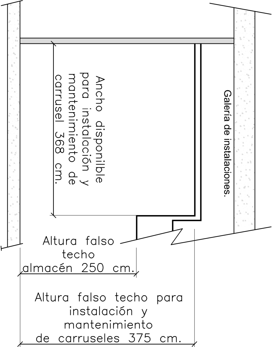
Sección C-C
