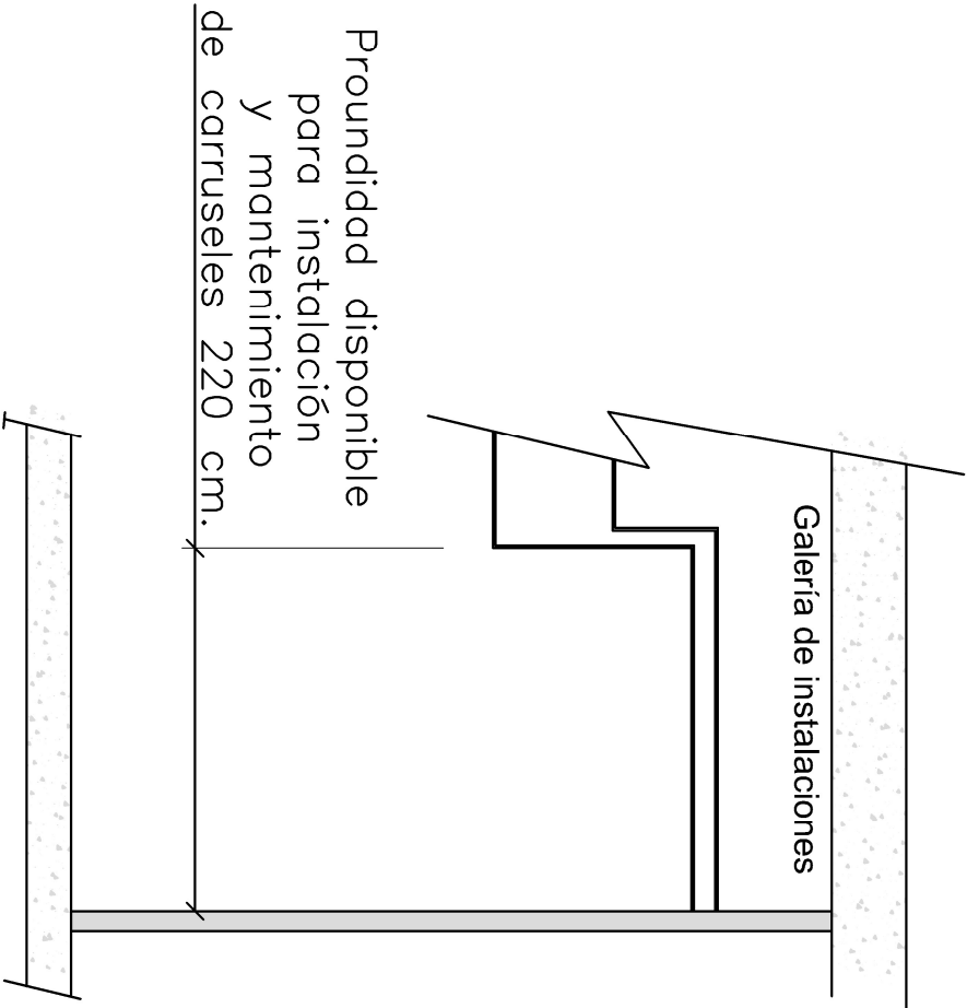
Sección D-D
