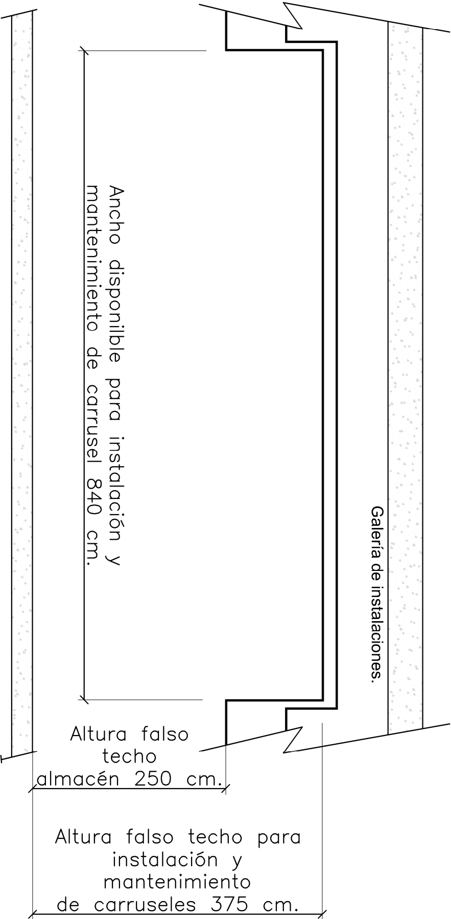
Sección A-A
