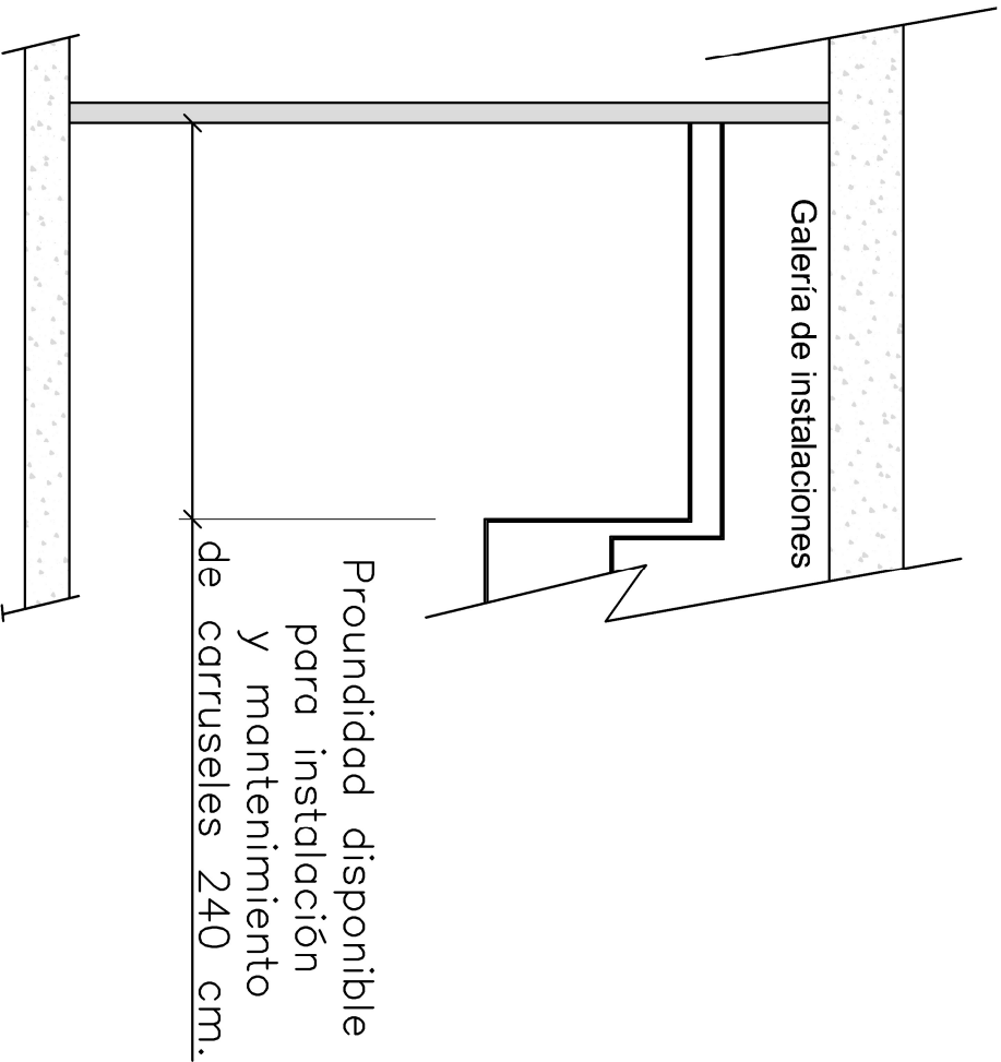
Sección B-B
