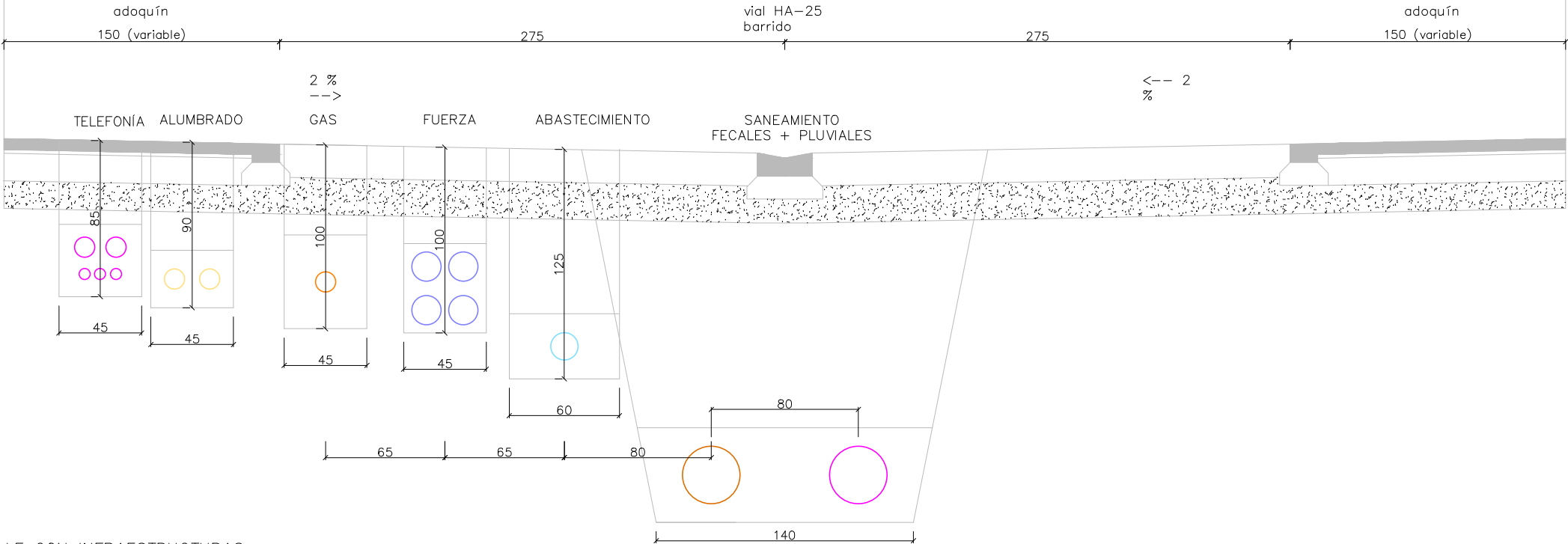
SECCIÓN TIPO DE CALLE CON INFRAESTRUCTURAS
