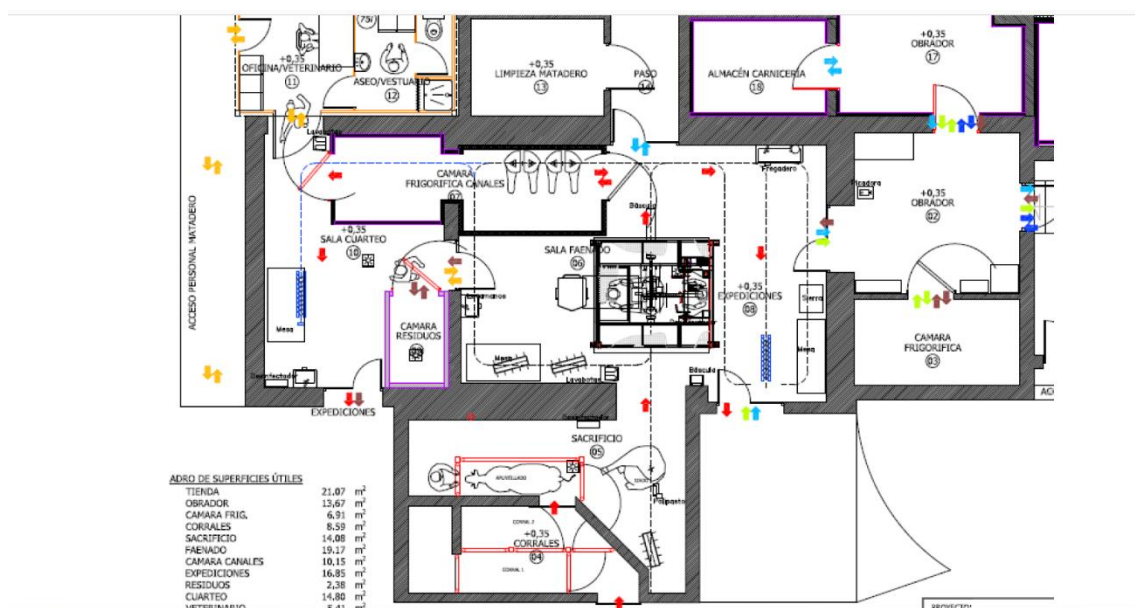
Imagen 10 Plano adecuación Matadero de Garralda y servicio carnicería
