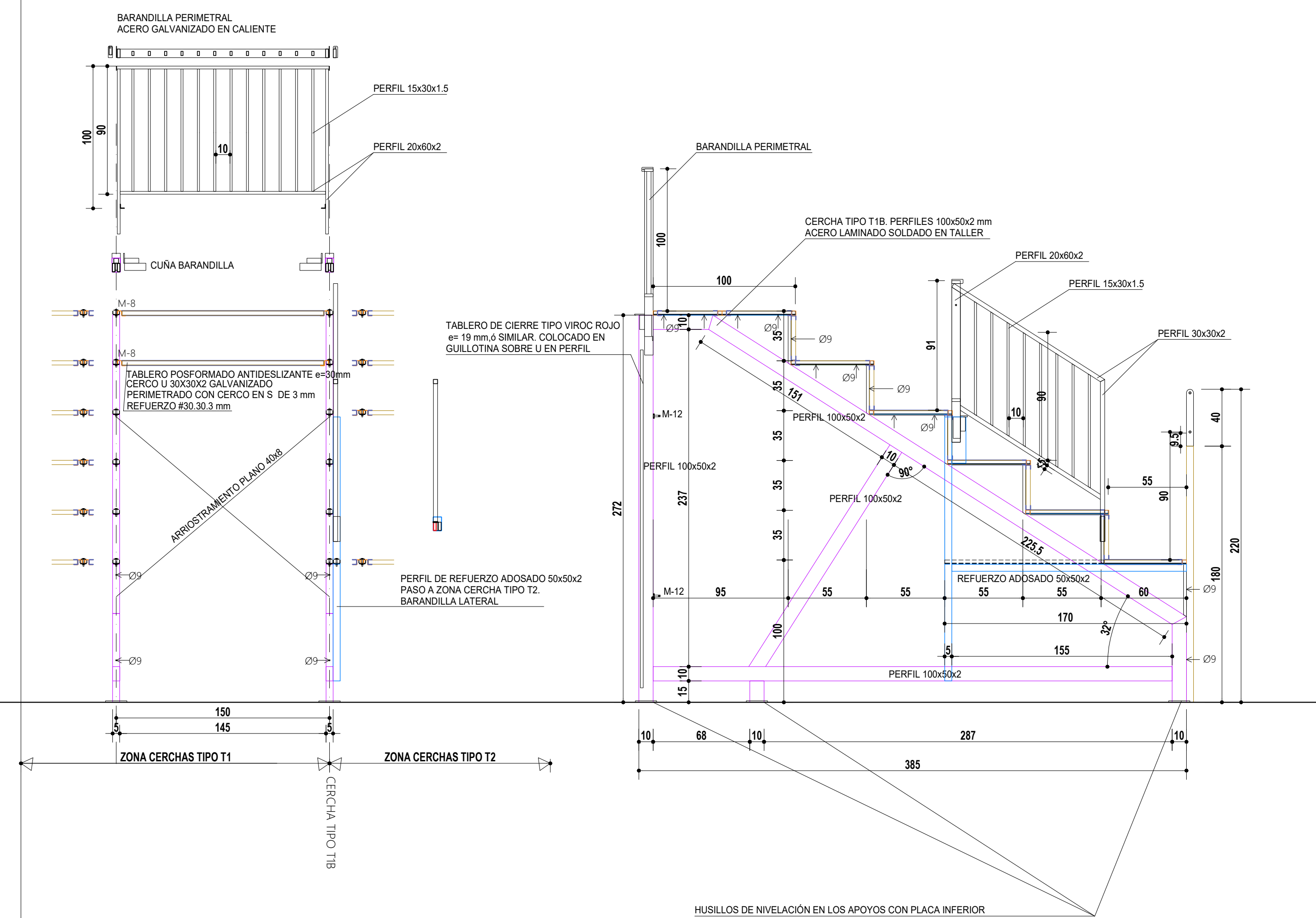
CERCHA TIPO T1B. BARANDILLA LATERAL
