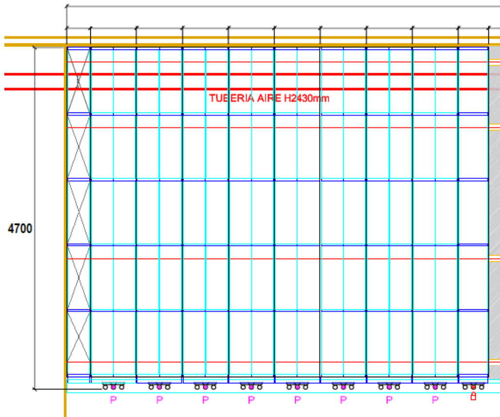
Gráfico 6b: Medidas de la envolvente de la planta (sin escala), con estanterías dibujadas (arqueta)
