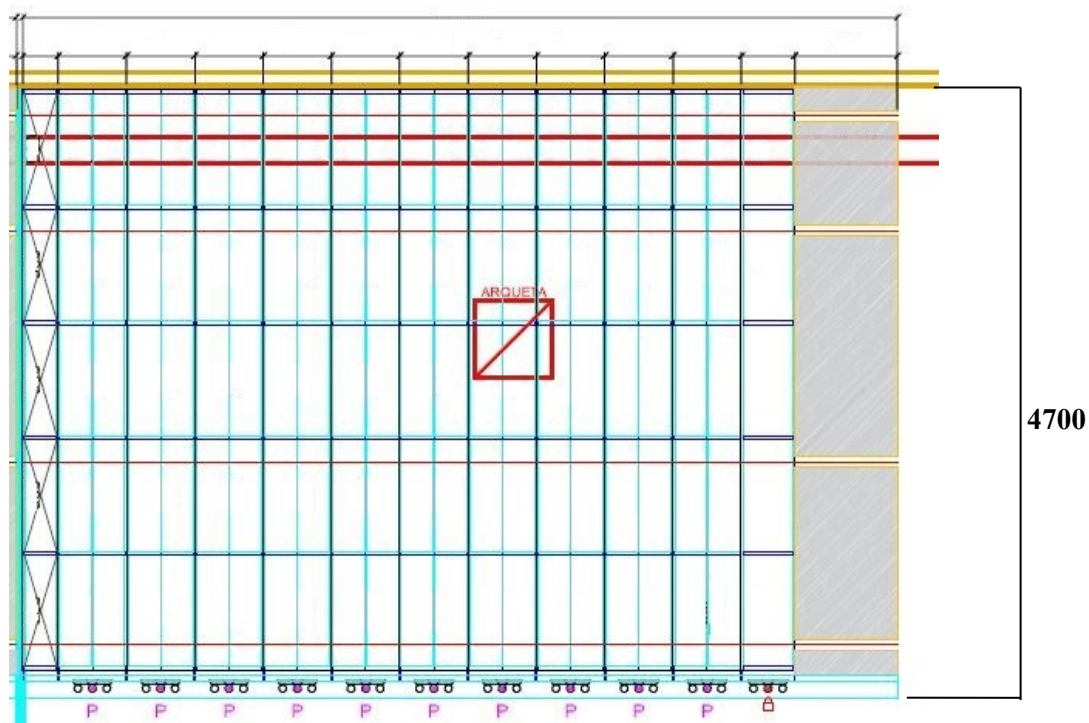
Gráfico 6b: Medidas de la envolvente de la planta (sin escala), con estanterías dibujadas (arqueta)
