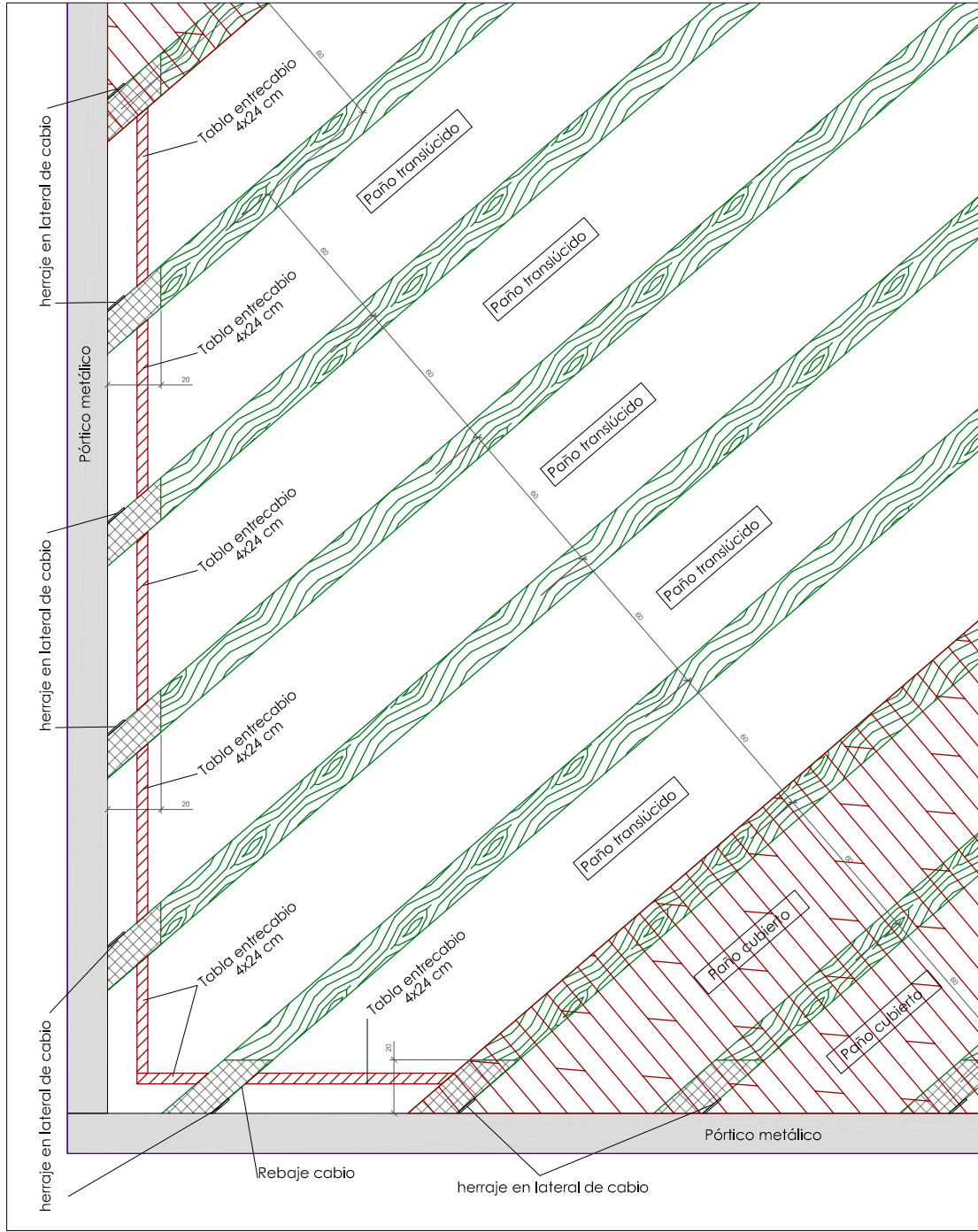
DETALLE CONSTRUCTIVO D-2. 1/20
