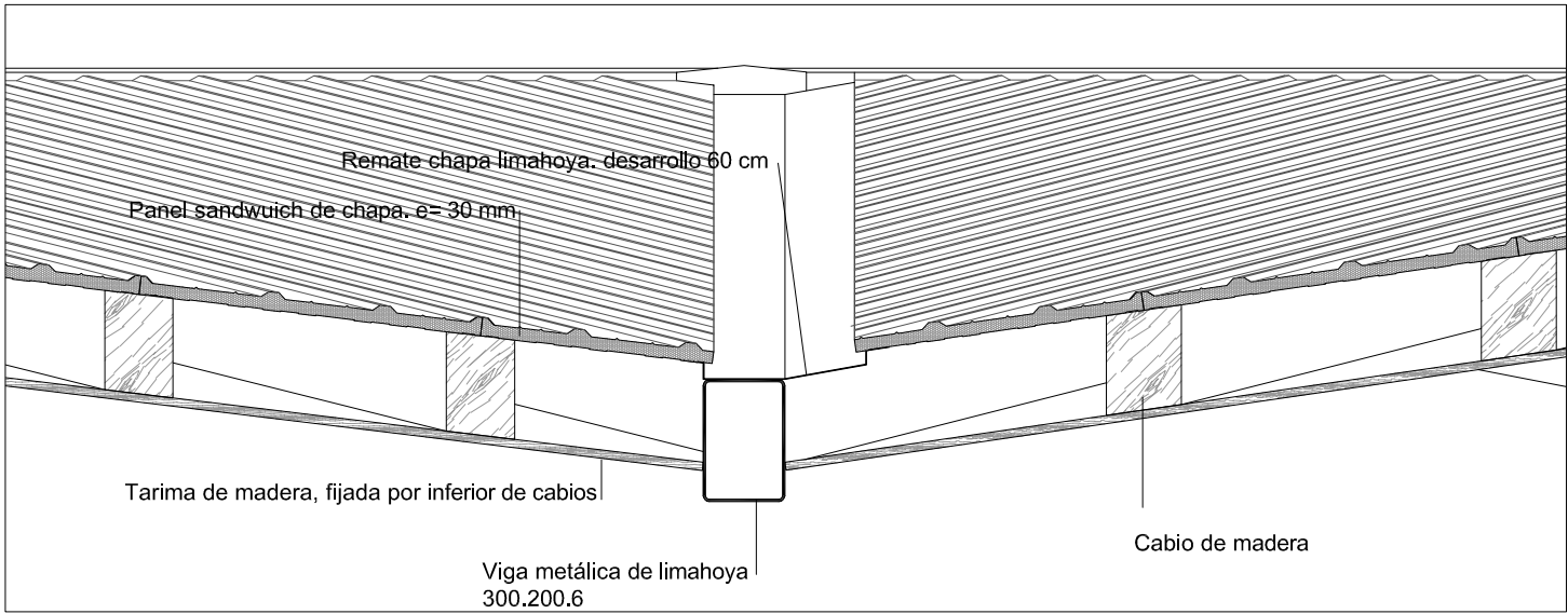
DETALLE CONSTRUCTIVO D-3. 1/20
