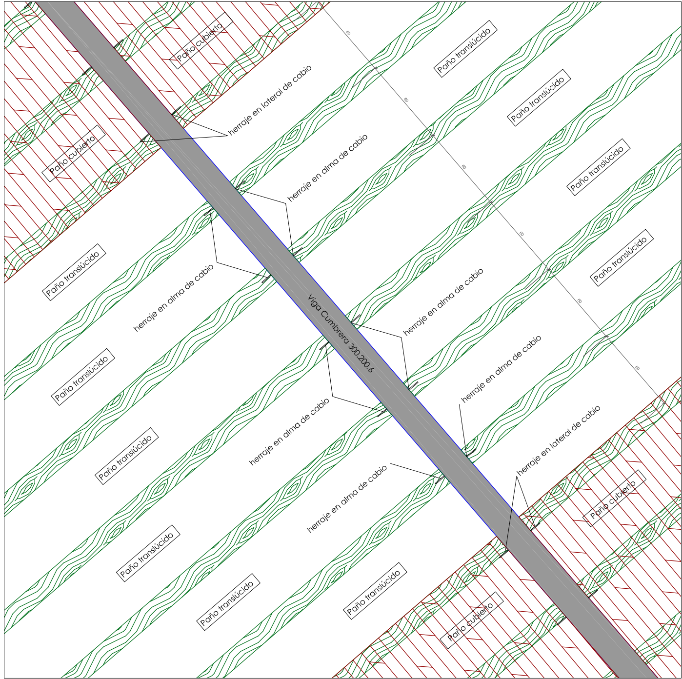
DETALLE CONSTRUCTIVO D-3. 1/20
