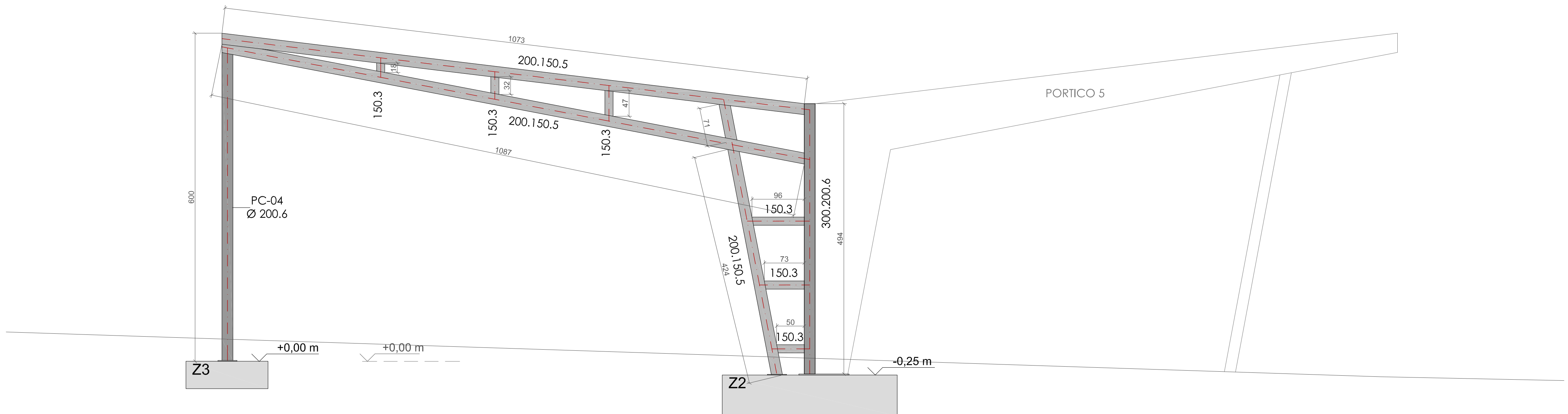
ALZADO PÓRTICO 4
