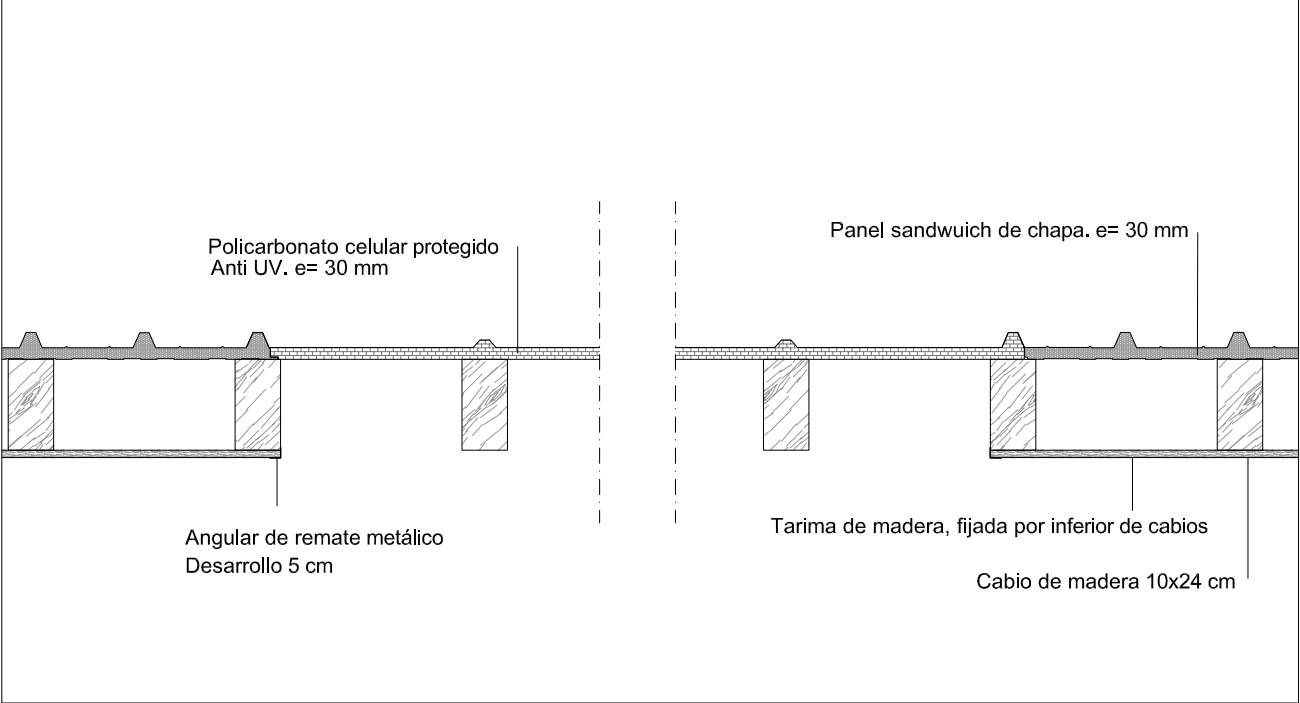
DETALLE CONSTRUCTIVO D-4. 1/20
