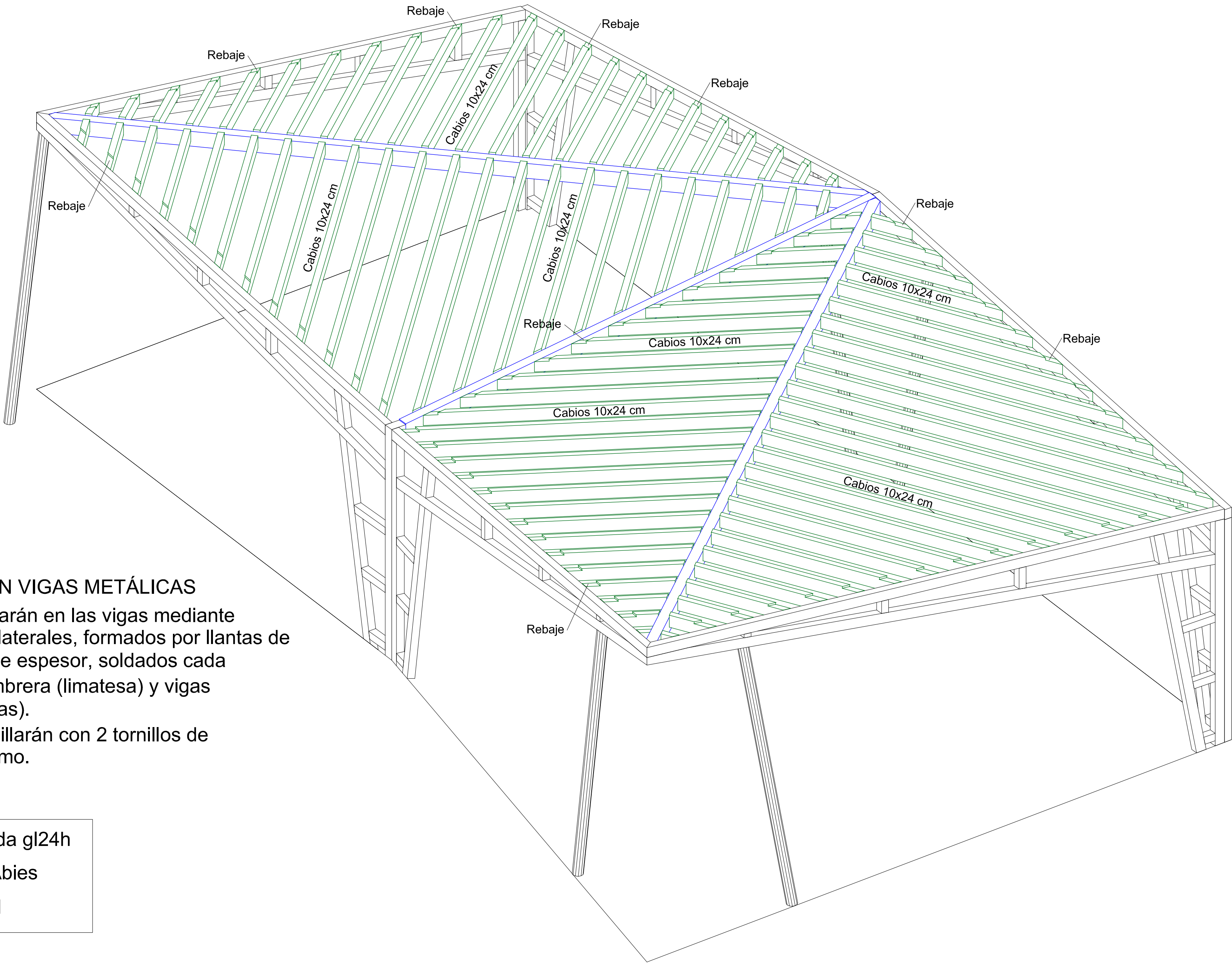
DETALLE D-2
