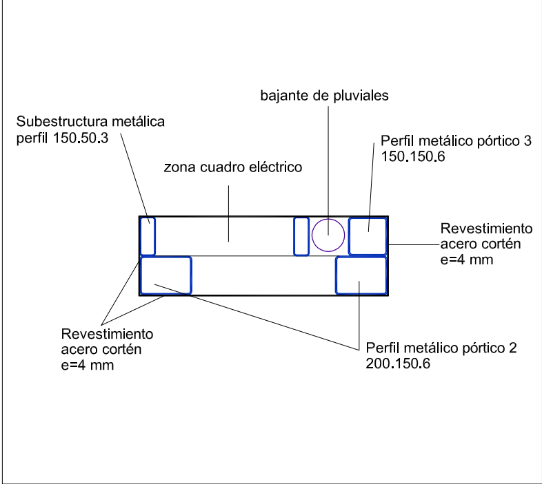
DETALLE HORIZONTAL DE PILAR PORTICO 2-3. 1/20
