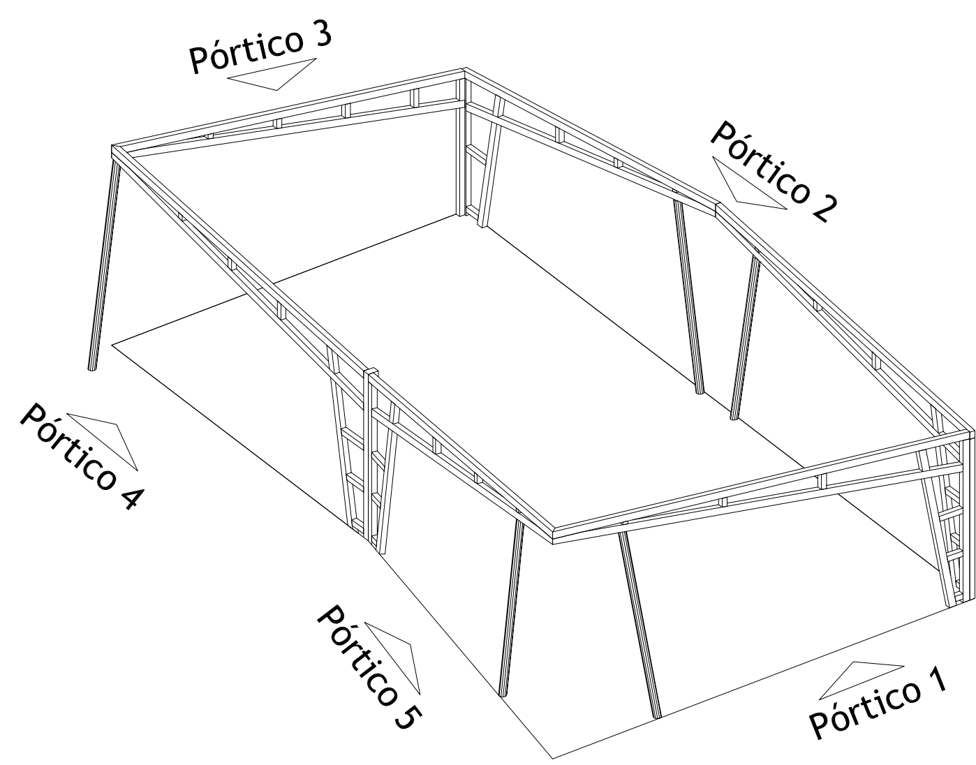
AXONOMÉTRICO POSICIÓN
