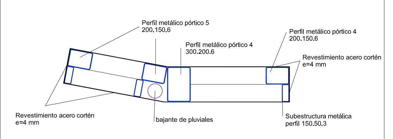
DETALLE HORIZONTAL DE PILAR PORTICO 4-5. 1/20
