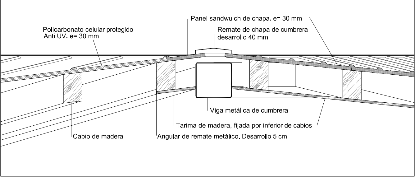
DETALLE CONSTRUCTIVO D-1. 1/20
