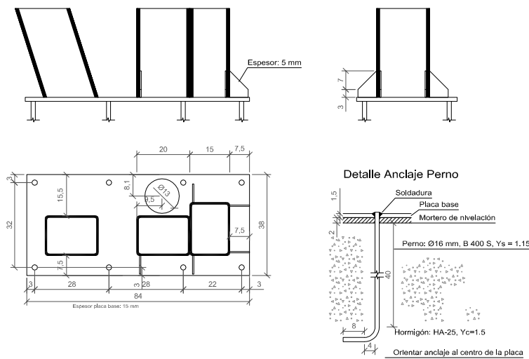
PLACA DE ANCLAJE P4 Placa. 84x38x1,5 cm
