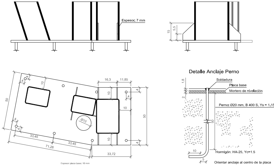
PLACA DE ANCLAJE P2 Placa. 104x50x1,8 cm
