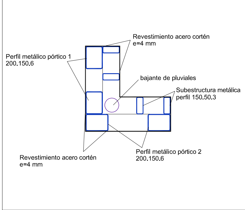
DETALLE HORIZONTAL DE PILAR PORTICO 1-2. 1/20
