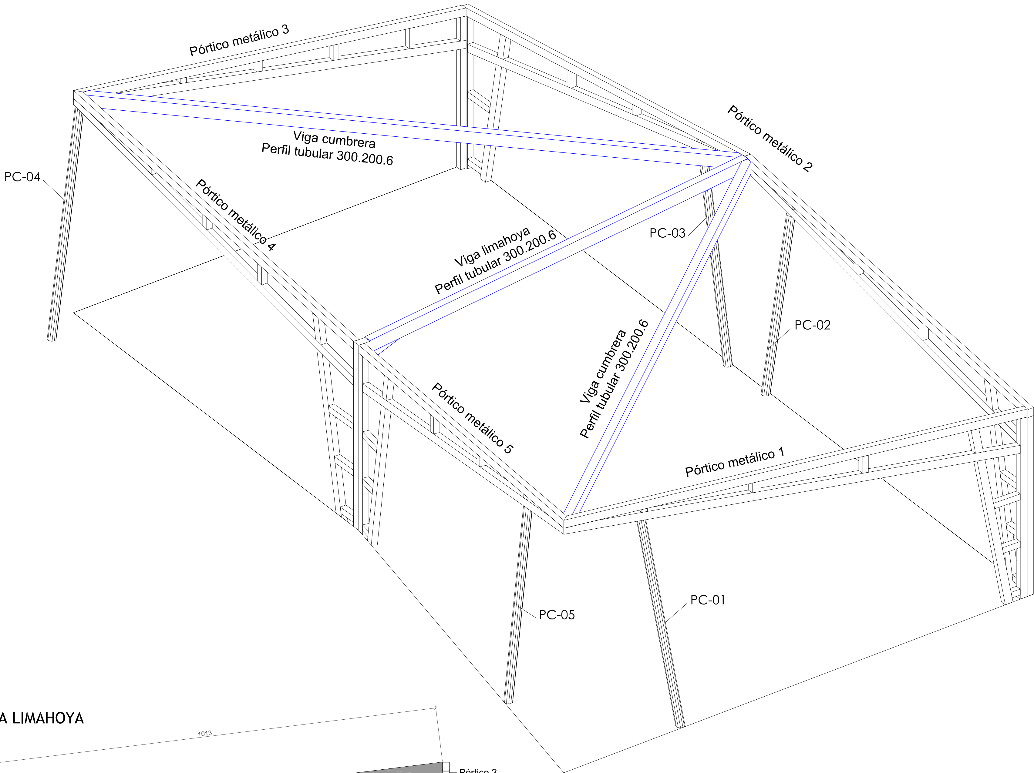
AXONOMÉTRICO DE ESTRUCTURA PRINCIPAL. VIGAS METÁLICAS
