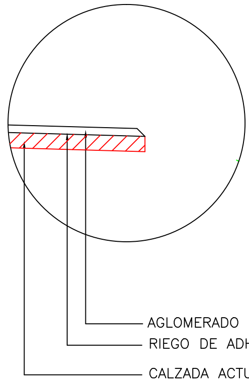
DETALLE A SECCION DE FIRME ESCALA 1:25
