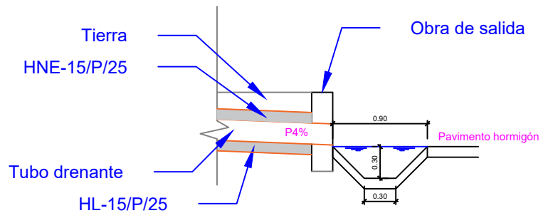
Sección llegada a obra de Drenaje Profundo
