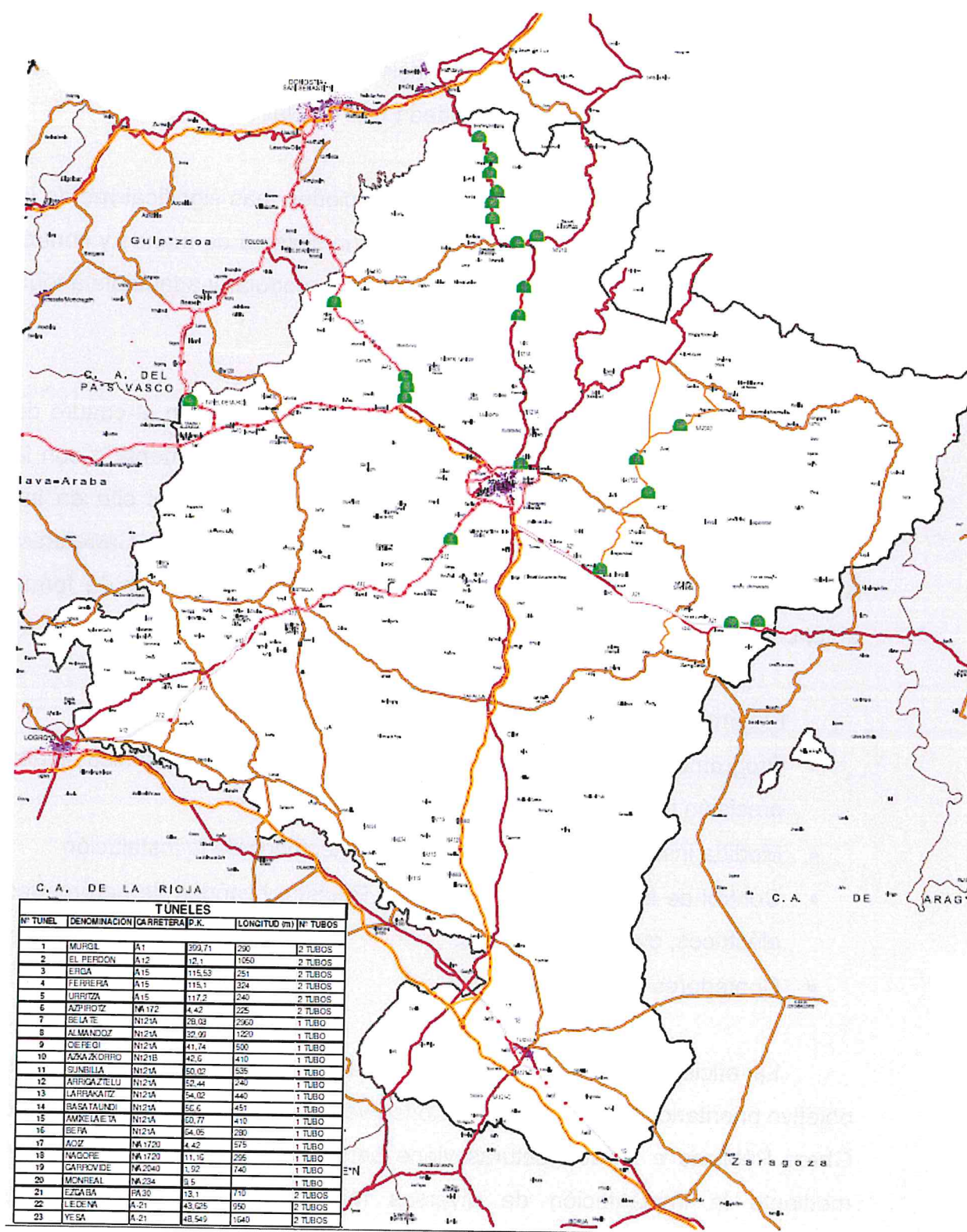
TUNELES EQUIPADOS EN LA RED DE CARRETERAS DEL GOBIERNO DE NAVARRA
