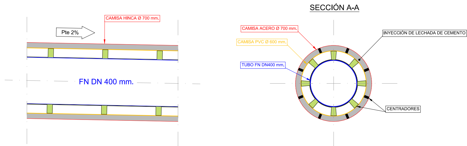
DETALLE DE PASO DE TUBO EN HINCA DE ACERO CON INYECCIÓN DE LECHADA DE CEMENTO
