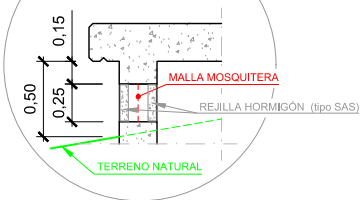
Sección B-B
