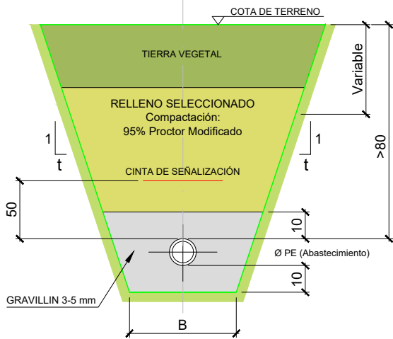
Zanja tipo acometida riego PE
