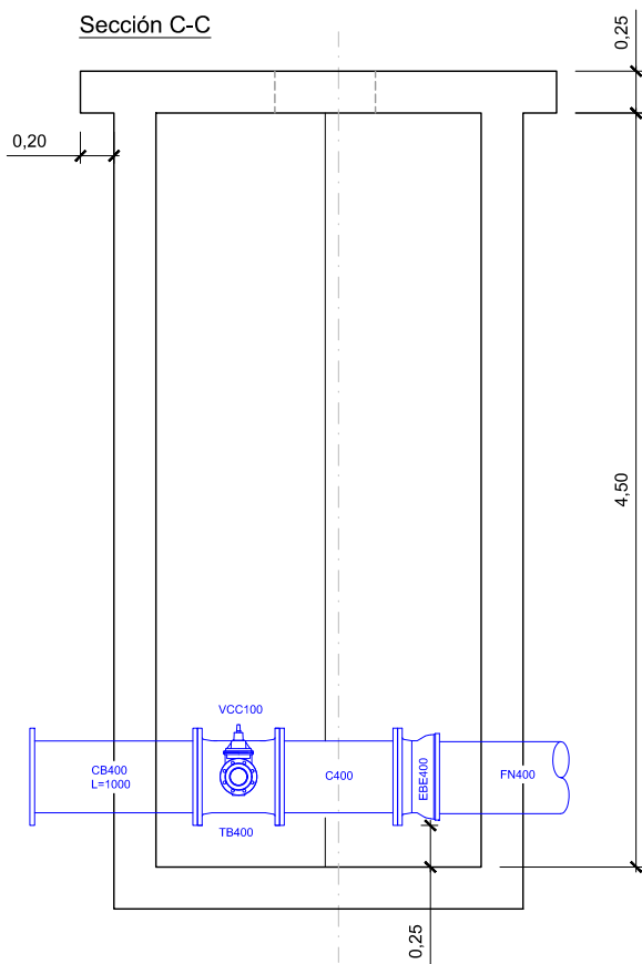
NUDO - D1
