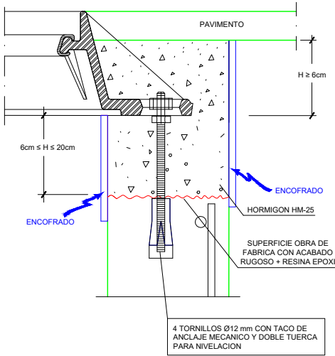
DETALLE 1 (FIJACIÓN DEL MARCO DE LAS TAPAS TIPO REXEL Y PAMREX). E=1/5
