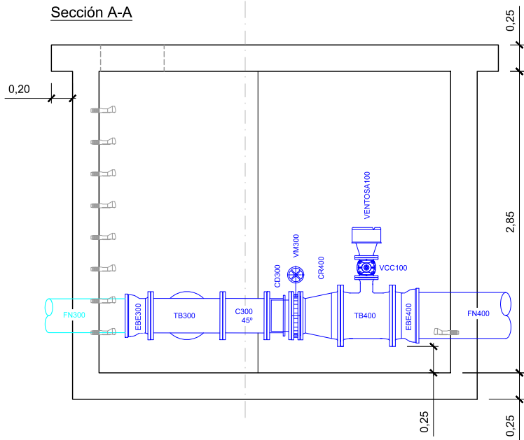
NUDO - C2
