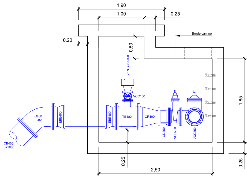
Sección D-D
