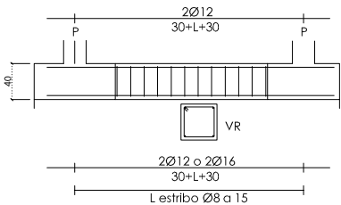
ESQUEMA VIGA RIOSTRA
