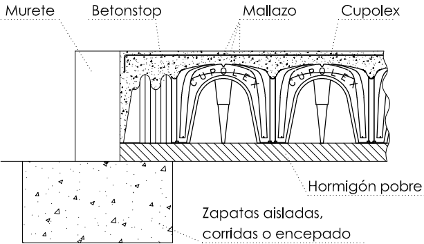
DETALLE GENÉRICO ENCUENTRO CON MURO
