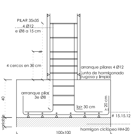
DETALLE ZAPATA - PILAR HORMIGON
