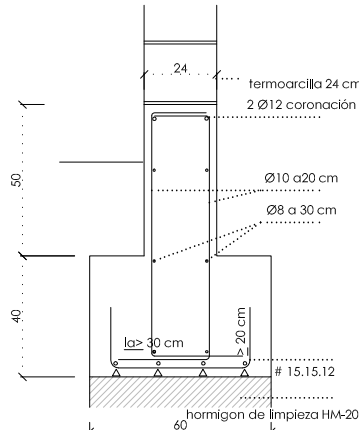
DETALLE ZAPATA CORRIDA
