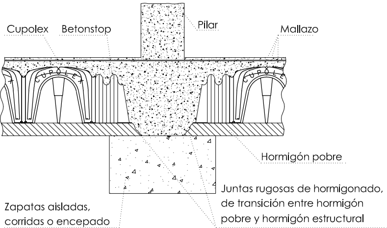
DETALLE GENÉRICO ENCUENTRO CON PILAR
