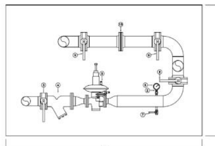
VISTA FRONTAL LINEAS TRASERAS
