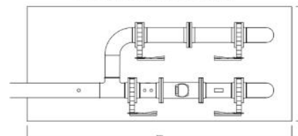
VISTA EN PLANTA UNIDAD DE MEDIDA
