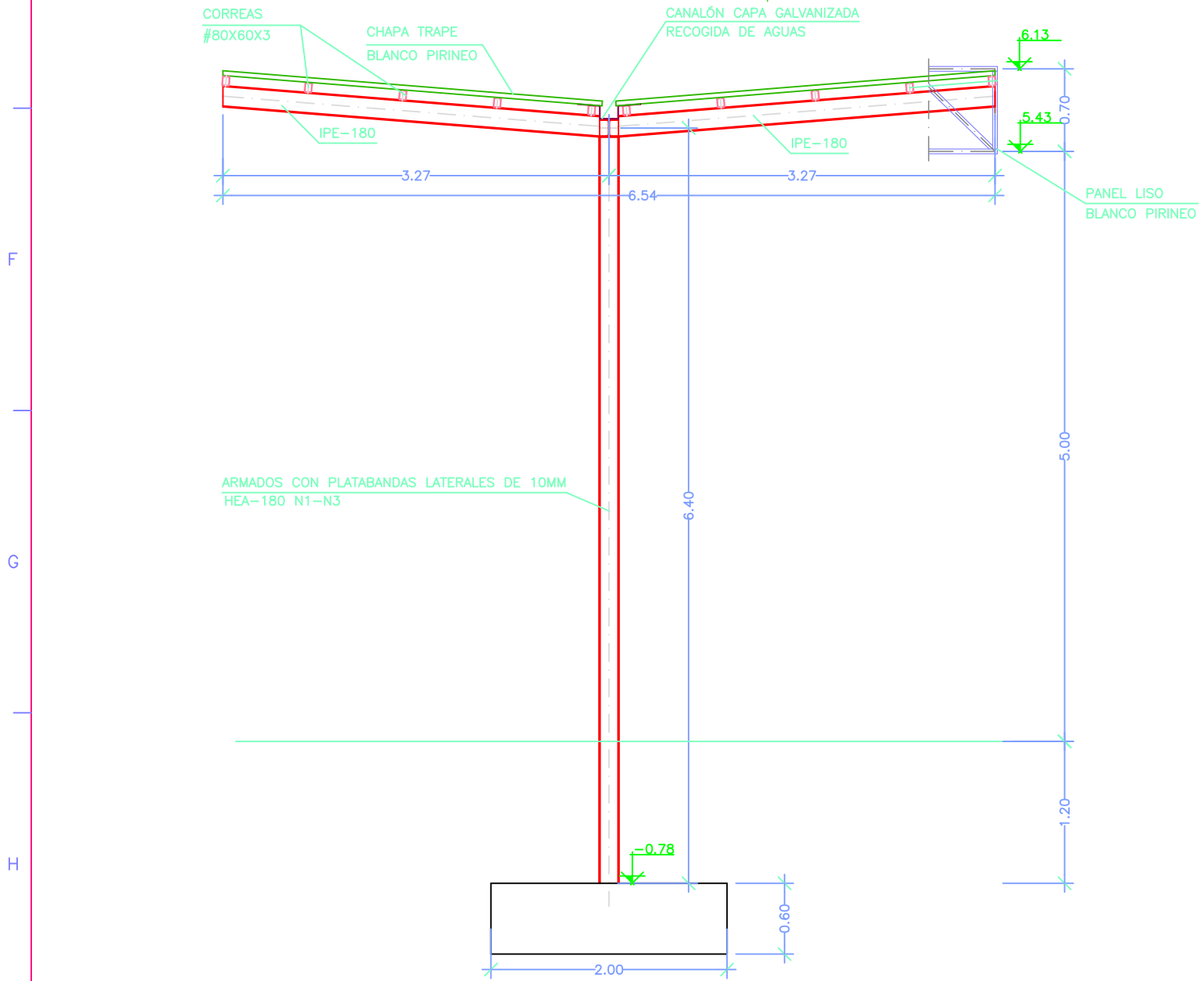
PORTICO 2 Y 3 ESCALA 1/50
