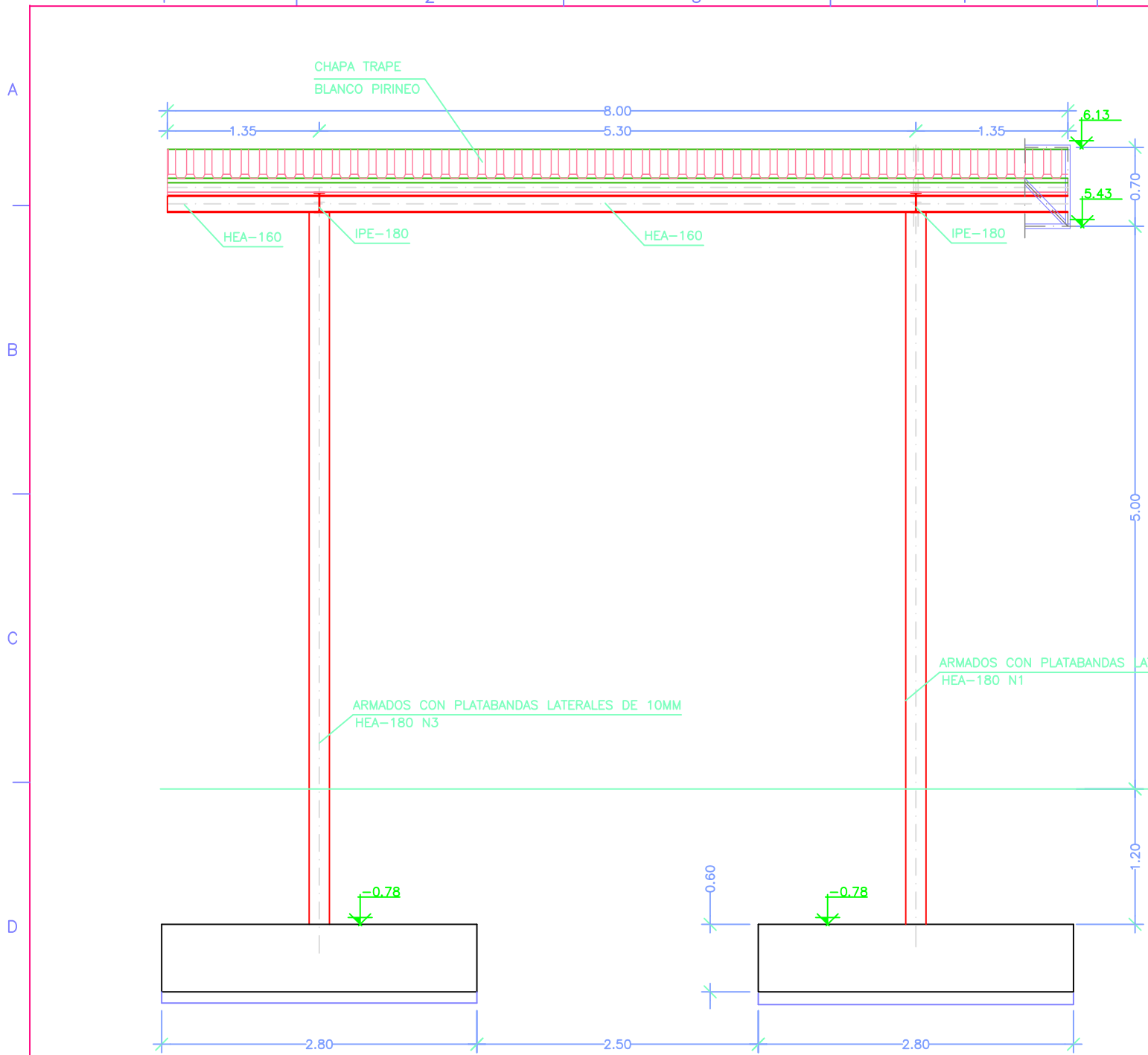
PORTICO 1 ESCALA 1/50
