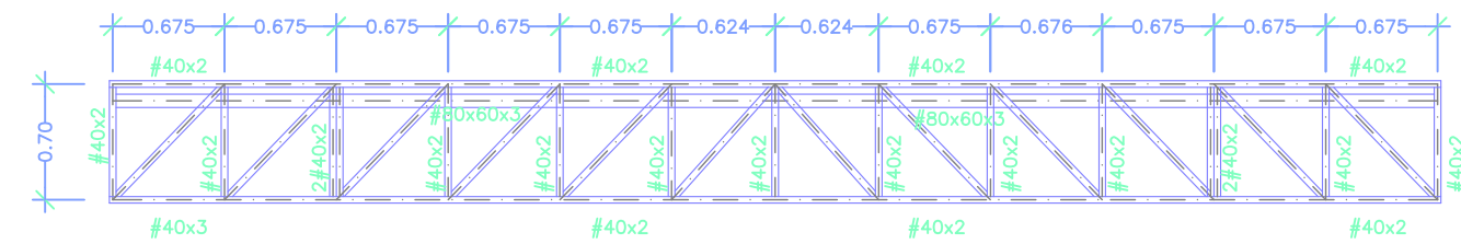
CERCHA 1 Y 3 ESCALA 1/50
