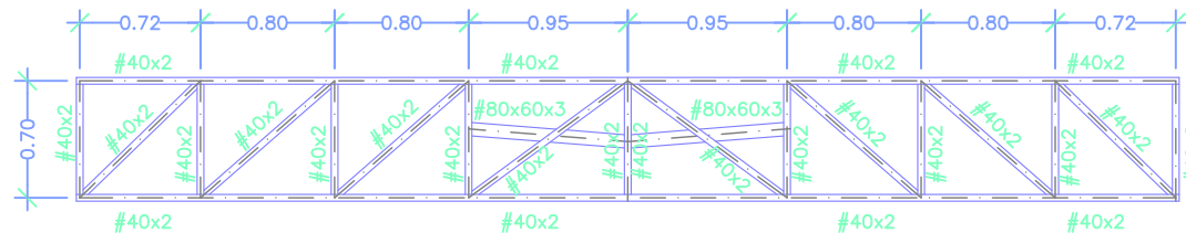
CERCHA 2 Y 4 ESCALA 1/50
