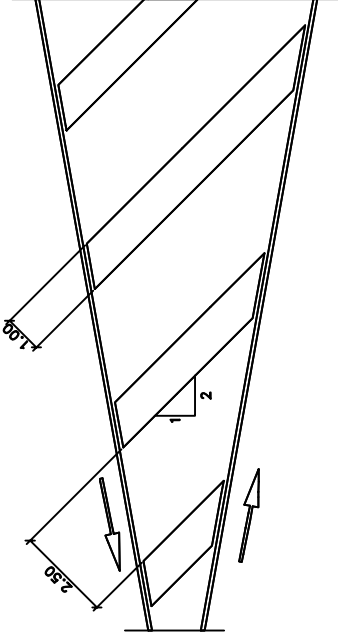
M-7.1.a VIA CON VM > 60 Km/h. CIRCULACION EN DOBLE SENTIDO
