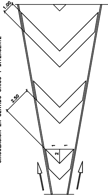
M-7.1.b VIA CON VM > 60 Km/h. CIRCULACION EN SENTIDO UNICO Y DIVERGENTE
