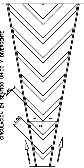
M-7.2.b VIA CON VM ≤ 60Km/h. CIRCULACION EN SENTIDO UNICO Y DIVERGENTE
