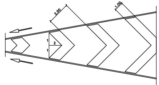
M-7.2.c VIA CON VM ≤ 60Km/h. CIRCULACION EN SENTIDO UNICO Y CONVERGENTE
