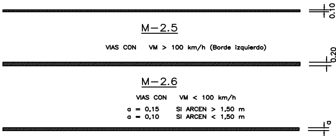
MARCAS LONGITUDINALES CONTINUAS ADOSADAS A DISCONTINUAS ESCALA : 1/100
