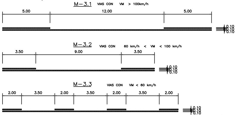
MARCAS TRANSVERSALES ESCALA : 1/100
