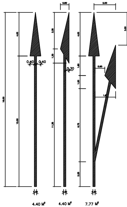
FLECHAS DE DIRECCION ESCALA 1/100 M-5-3
