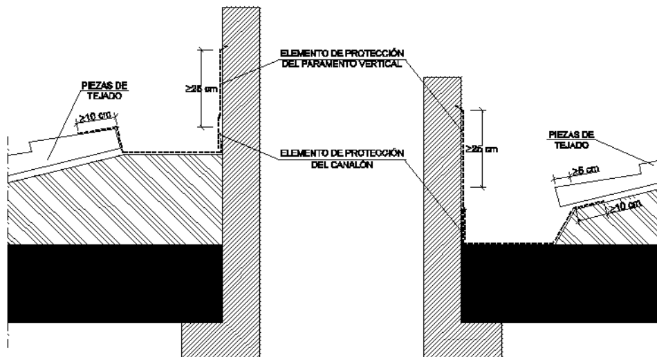
Figura 2.17 Canalones
