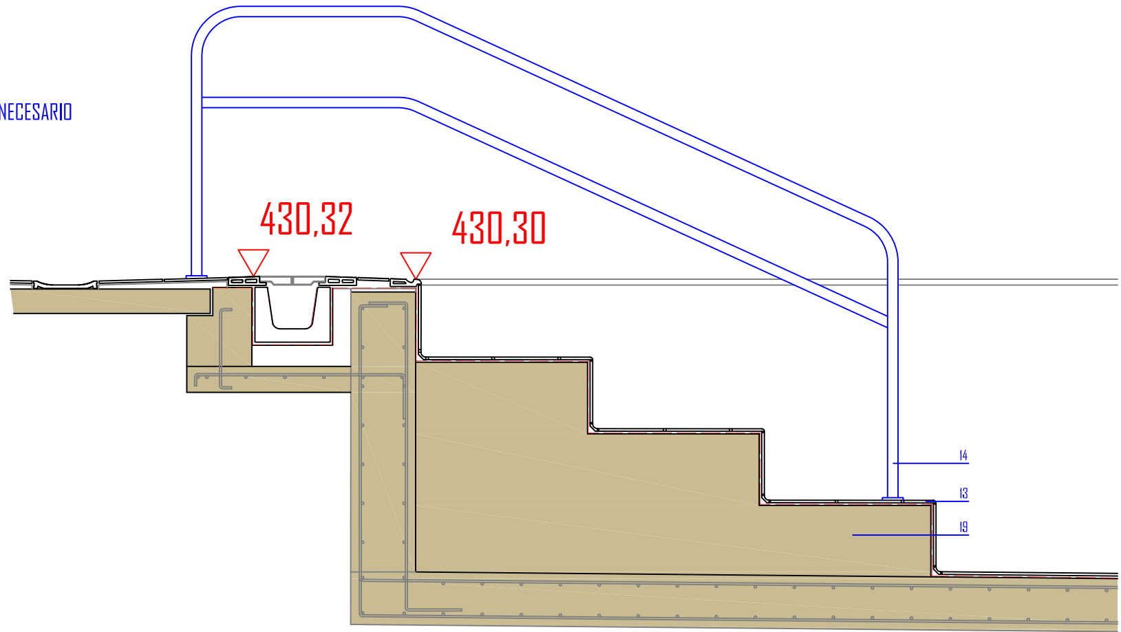
DETALLE CONSTRUCTIVO ESTADO REFORMADO
