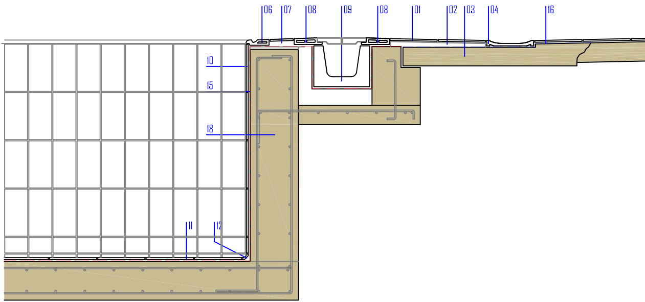
DETALLE CONSTRUCTIVO ESTADO REFORMADO
