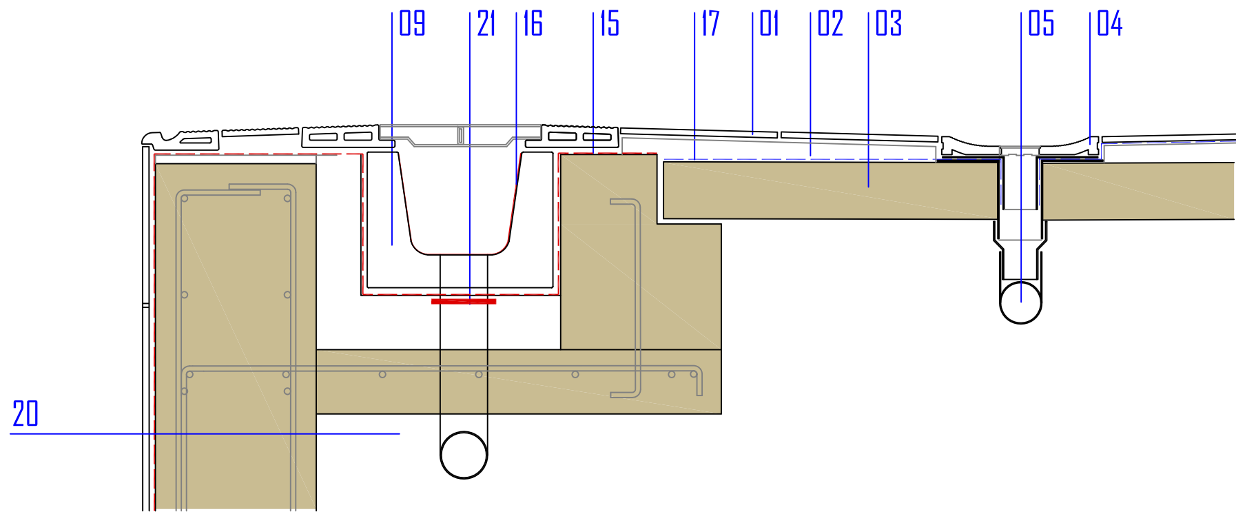
DETALLE CONSTRUCTIVO
