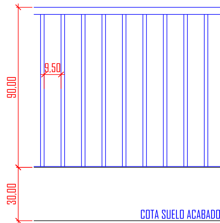
MURO CERRAMIENTO PLAYA
