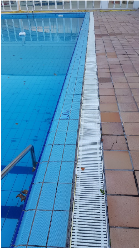
Vista borde piscina y rebosadero
