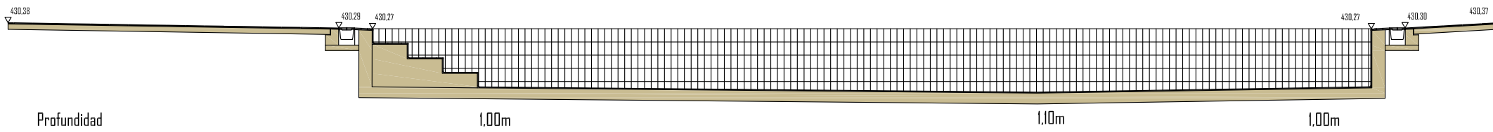
SECCIÓN BB
