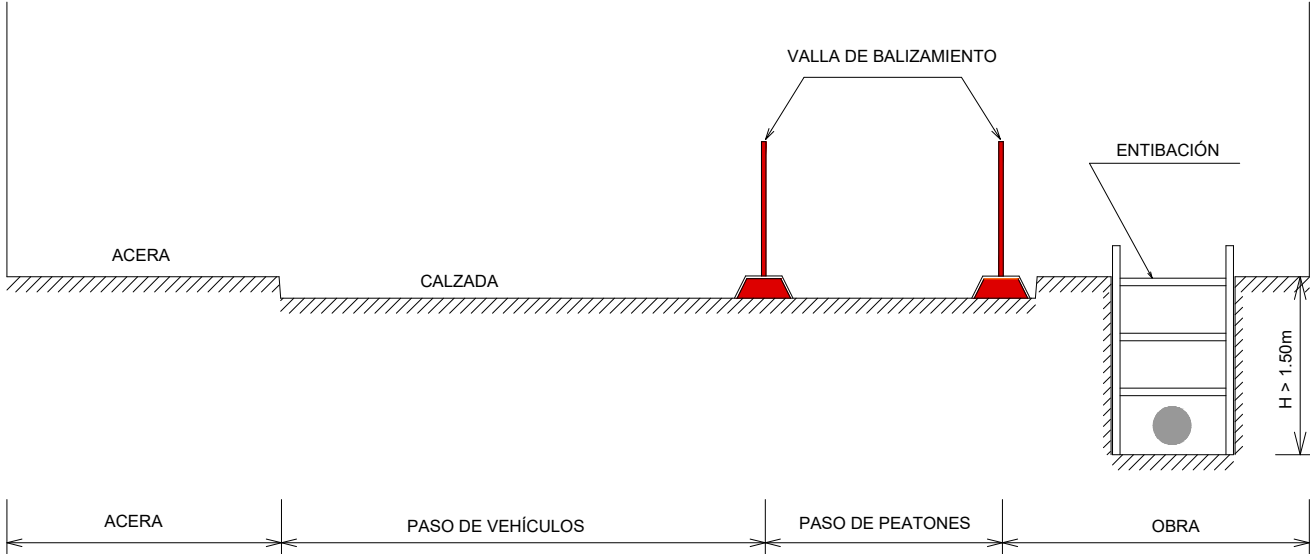
APERTURA DE ZANJA CON ENTIBACIÓN EN ACERA
