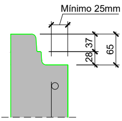
DETALLE - A (cotas en mm)
