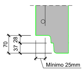
DETALLE - B (cotas en mm)
