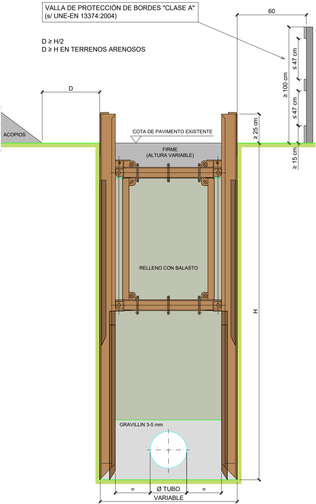
ZANJA TIPO ENTIBADA. E=1/20
