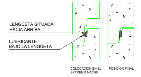
DETALLE DE LA JUNTA ENTRE MÓDULOS E=1/10
