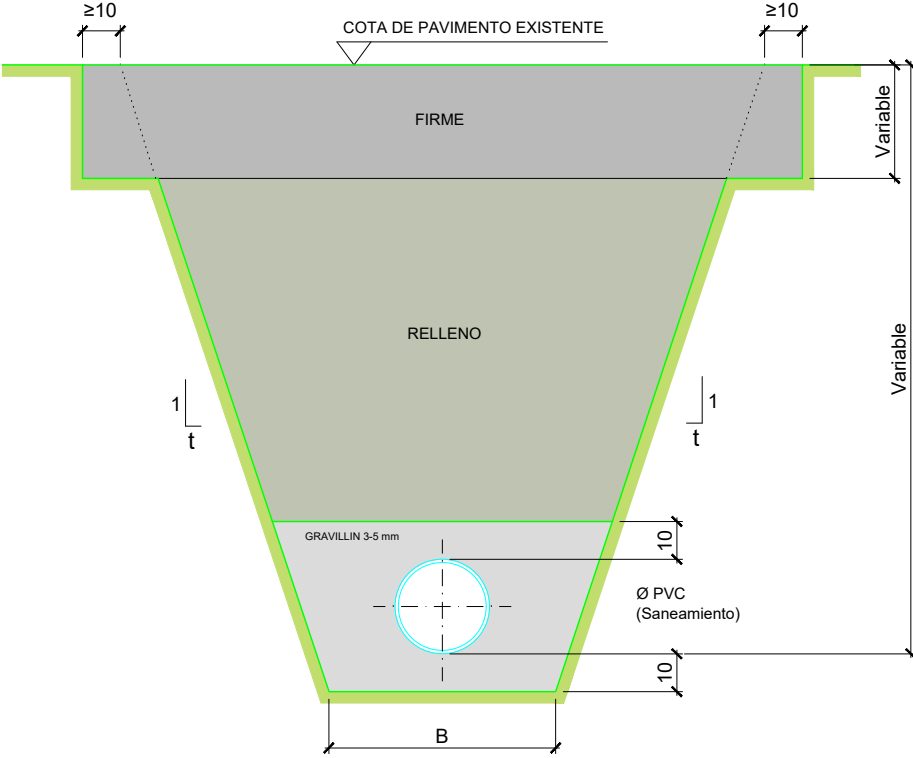
ZANJA TIPO SANEAMIENTO. E=1/20
