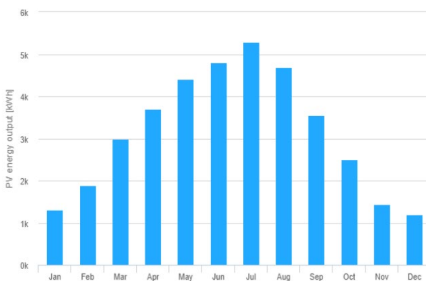
Gráfica 12: Producción fotovoltaica estimada cubierta oeste
