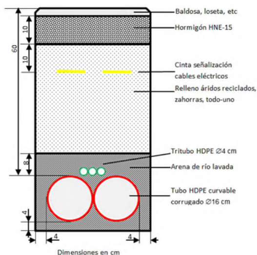
Ilustración 18: Distancias mínimas de la canalización a realizar
