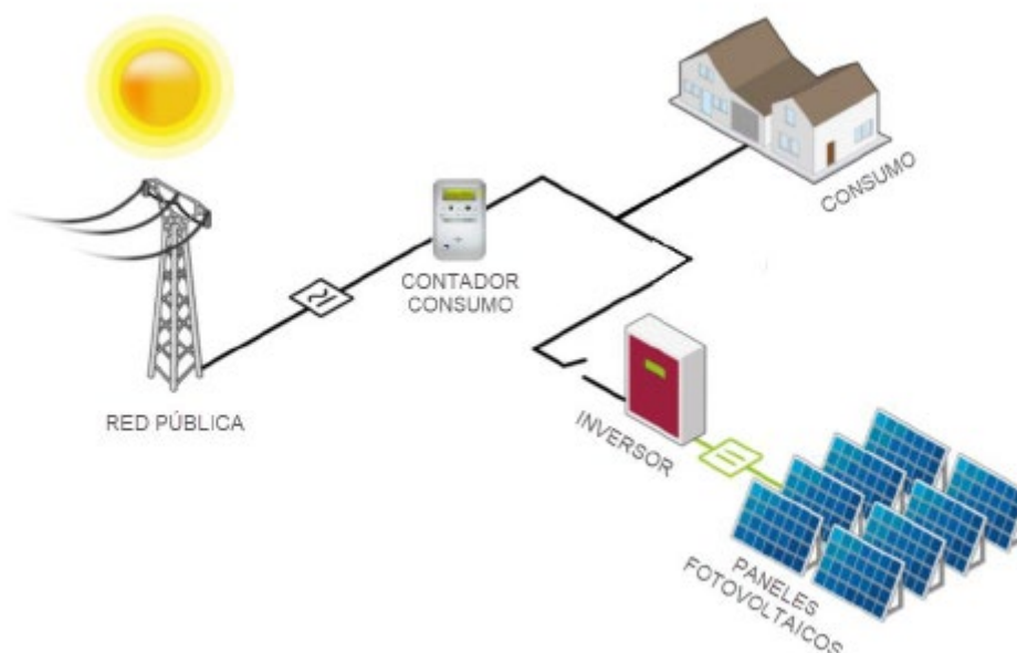
Ilustración 1: Esquema de una instalación fotovoltaica para autoconsumo
