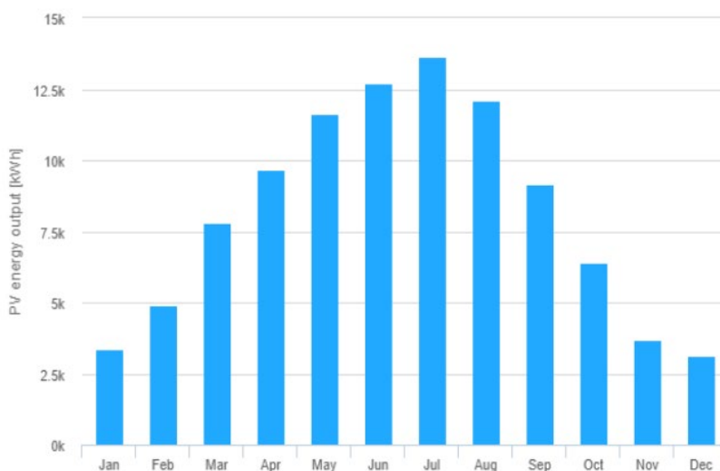
Ilustración 13. Producción fotovoltaica estimada cubierta este
