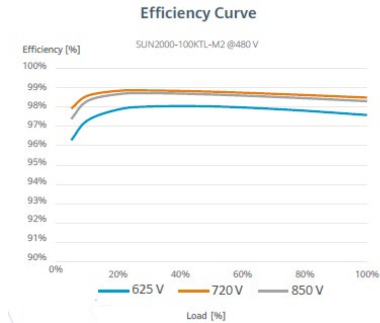
Ilustración 7: Curva de rendimiento del inversor
