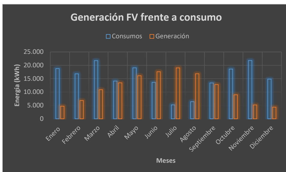
Ilustración 15. Generación fotovoltaica & Consumo total
