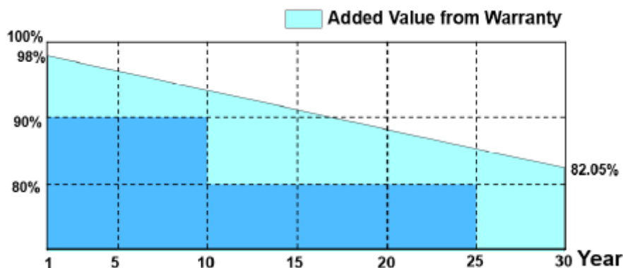
Ilustración 5: Variación de la potencia con el tiempo
