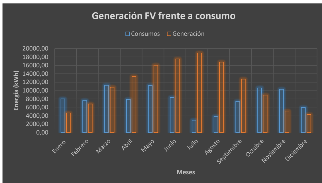
Gráfica 2: Generación fotovoltaica & Consumo colegio
