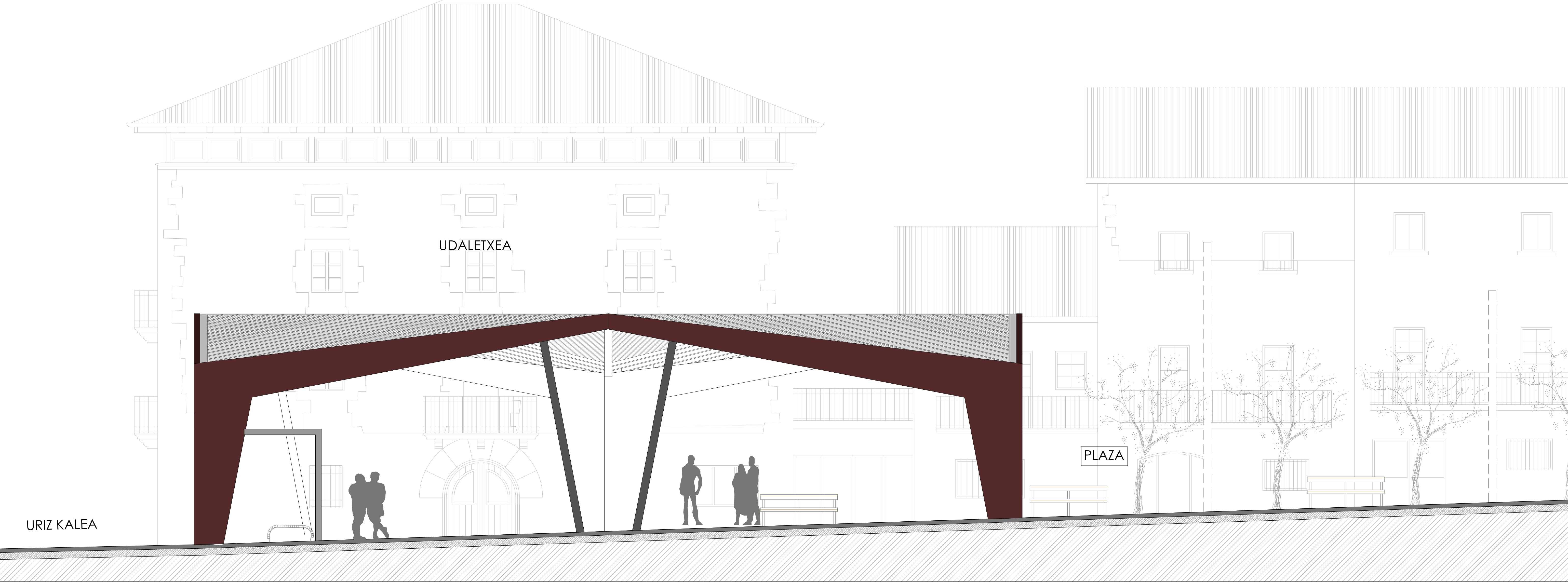
ALZADO OESTE
