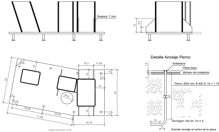
PLACA DE ANCLAJE P2 Placa. 104x50x1,8 cm
