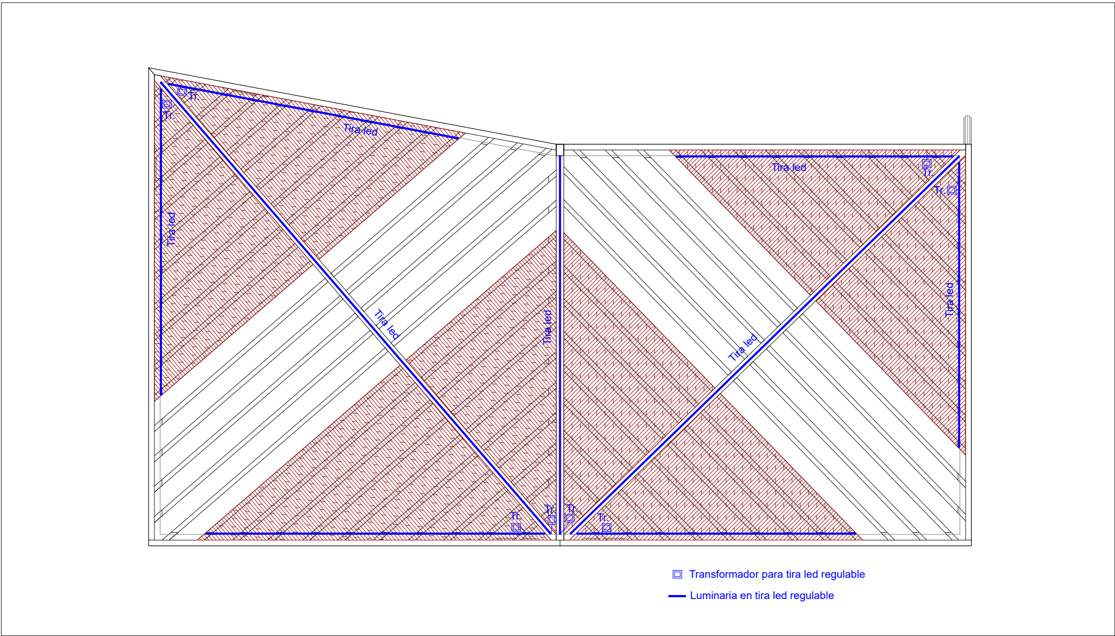
PLANTA DE LUMINARIAS
