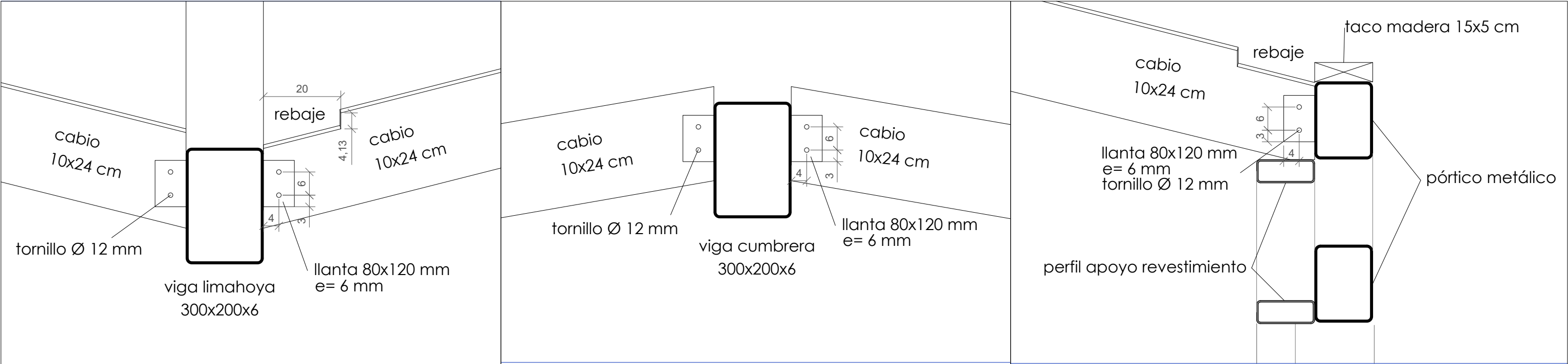
DETALLE D-1
