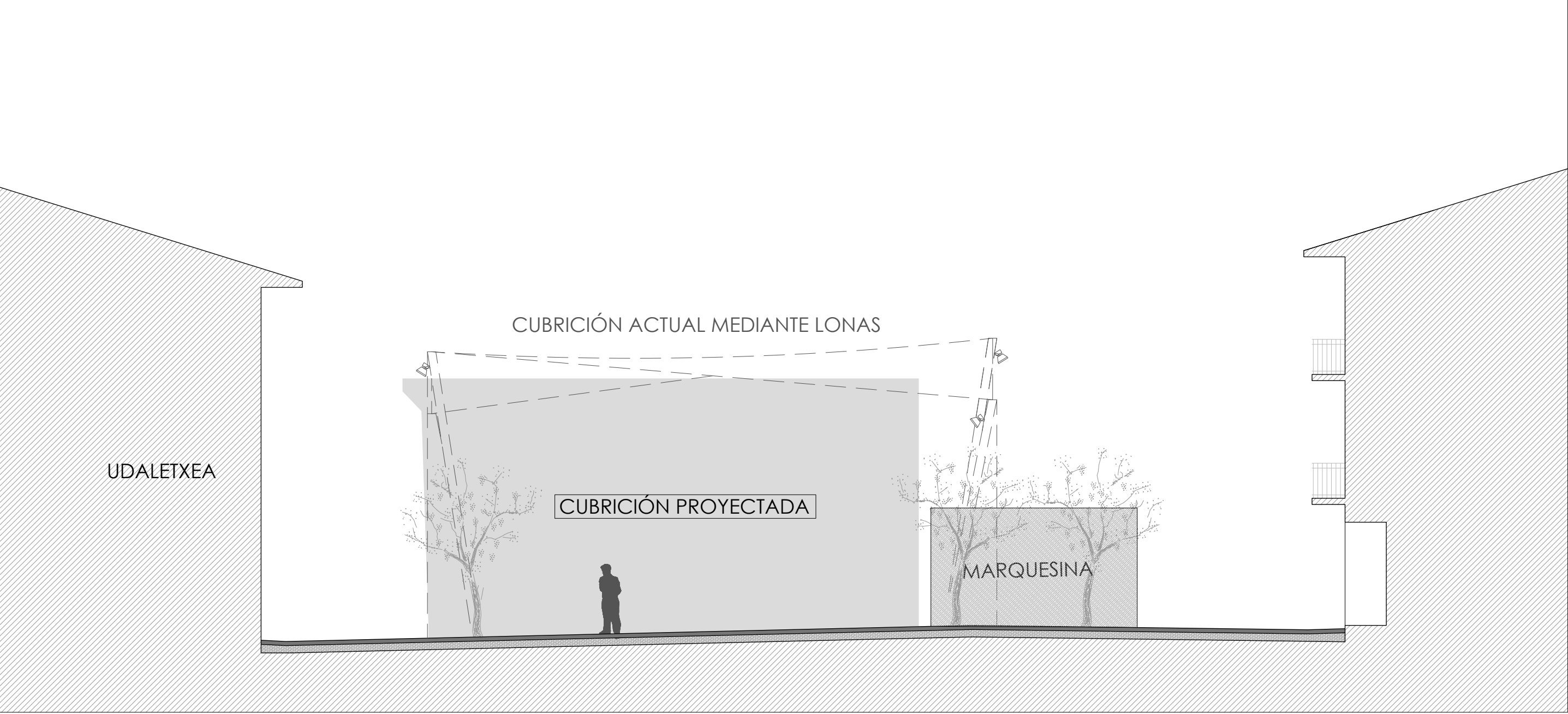
SECCIÓN TRANSVERSAL B-B
