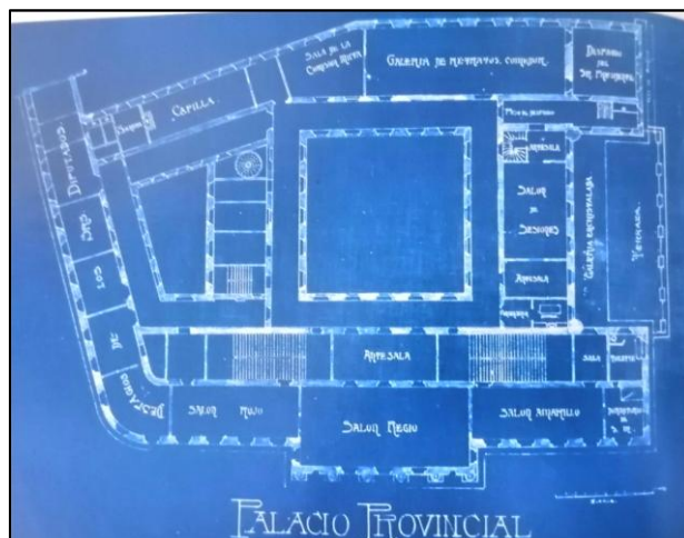
Fig. 63.- Plano de la planta principal del Palacio Provincial. 1851. (LARUMBE, 1990: 374; AGN)
