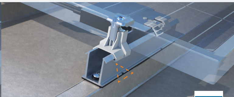
PERFIL DE MONTAJE PREPARADO PARA OPTIMIZADORES DE POTENCIA PARA INSTALACIÓN CON OPTIMIZADORES DE POTENCIA GR
