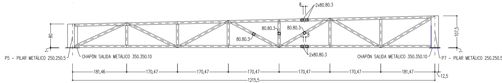
CERCHA 2
