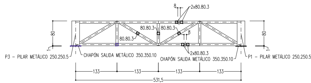
CERCHA 4
