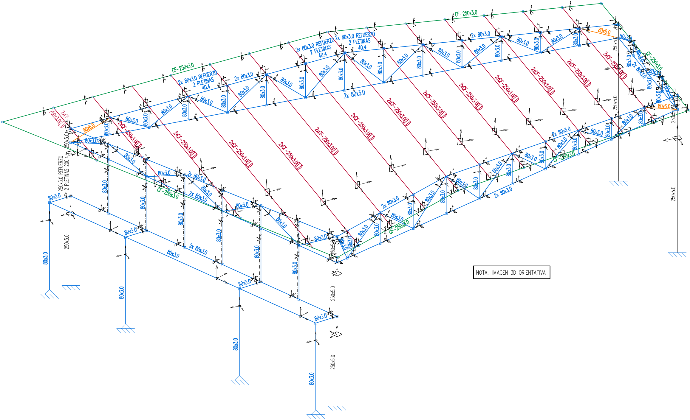
ESQUEMA 3D ALÁMBRICA
