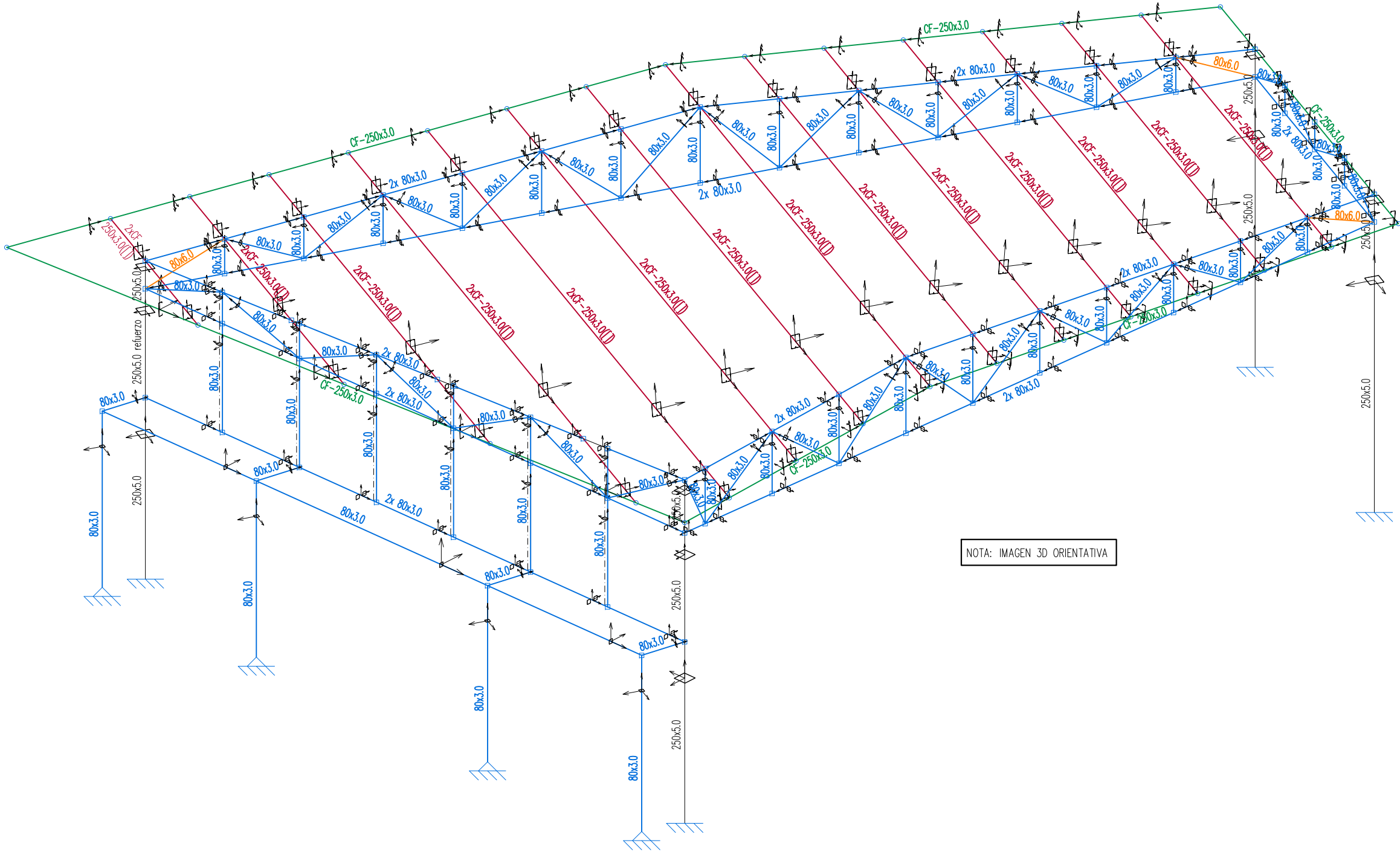
ESQUEMA 3D INALAMBRICO
