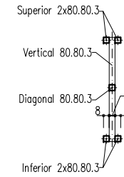
SECCIÓN TIPO CERCHAS
