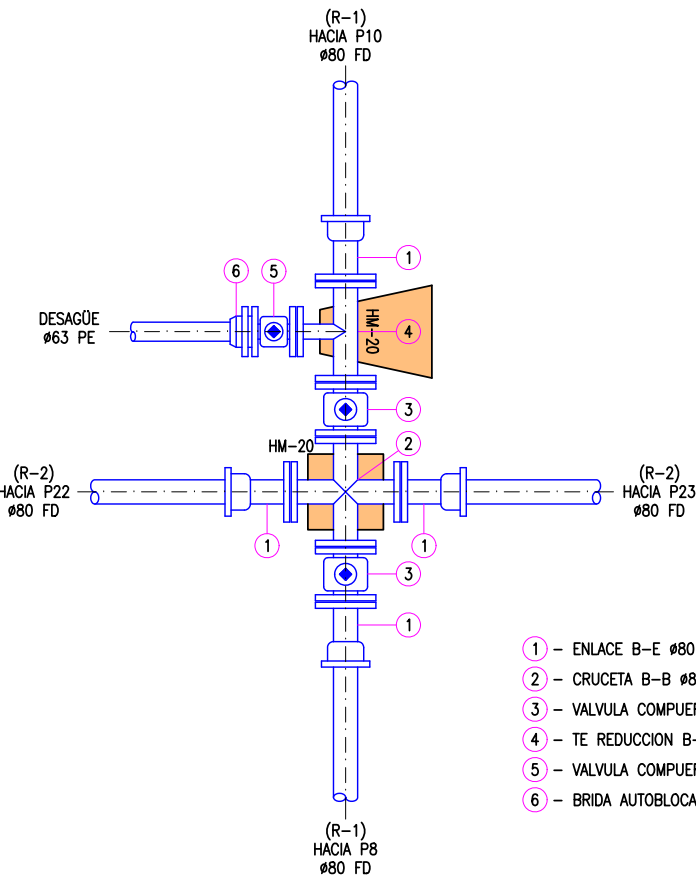
NUDO B
