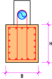
SECCION TRANSVERSAL
