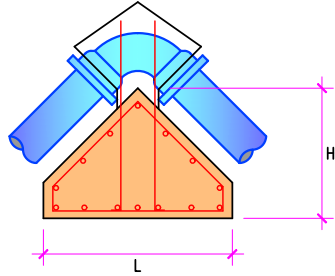
SECCION LONGITUDINAL
