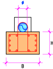
SECCION TRANSVERSAL
