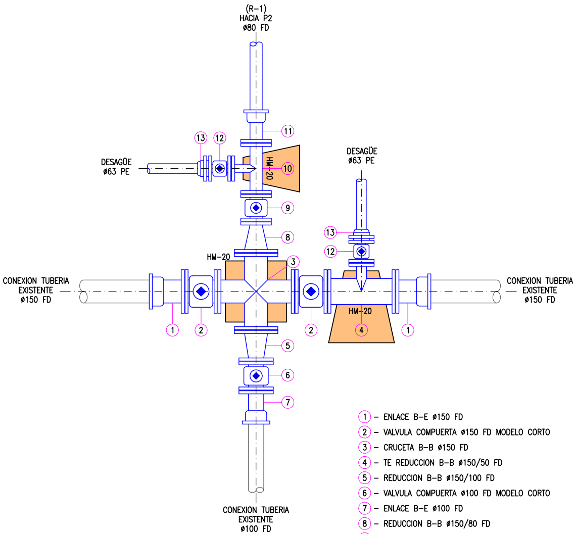
NUDO A
