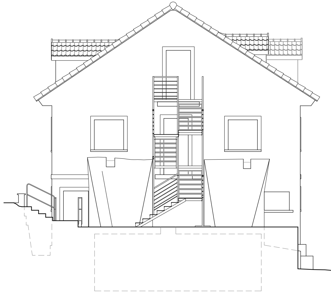
Alzado oeste
