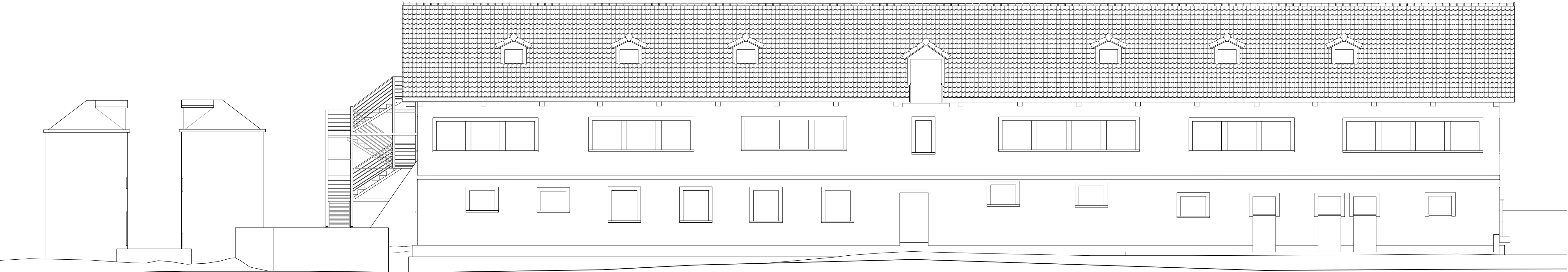
Alzado sur
