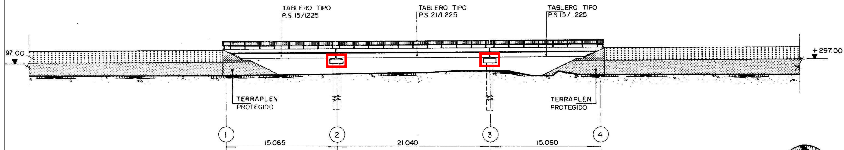
ALZADO (CALZADA DERECHA) ESCALA 1:250
