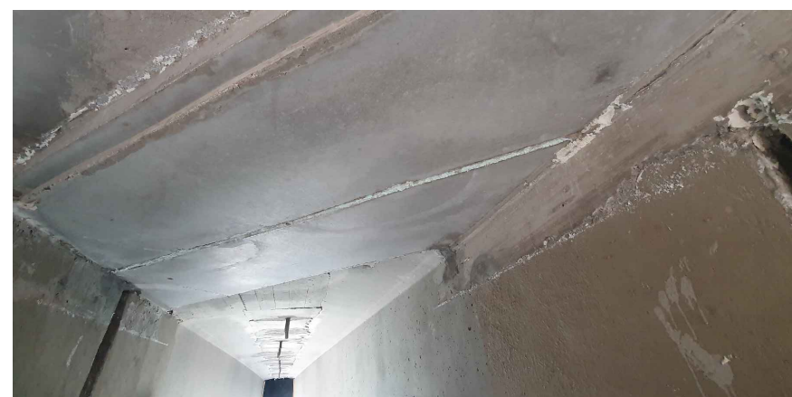
RECONSTRUCCIÓN DE ESTRUCTURAL LABIOS JUNTAS (INFERIOR)
