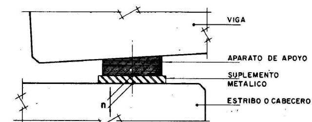
ESQUEMA DE APARATO DE APOYO (SECCION POR EJE DE VIGA)
