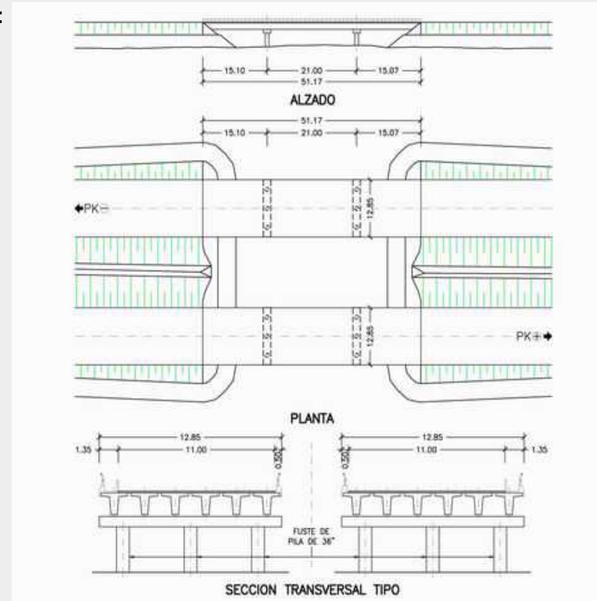
02-Alzado sur
