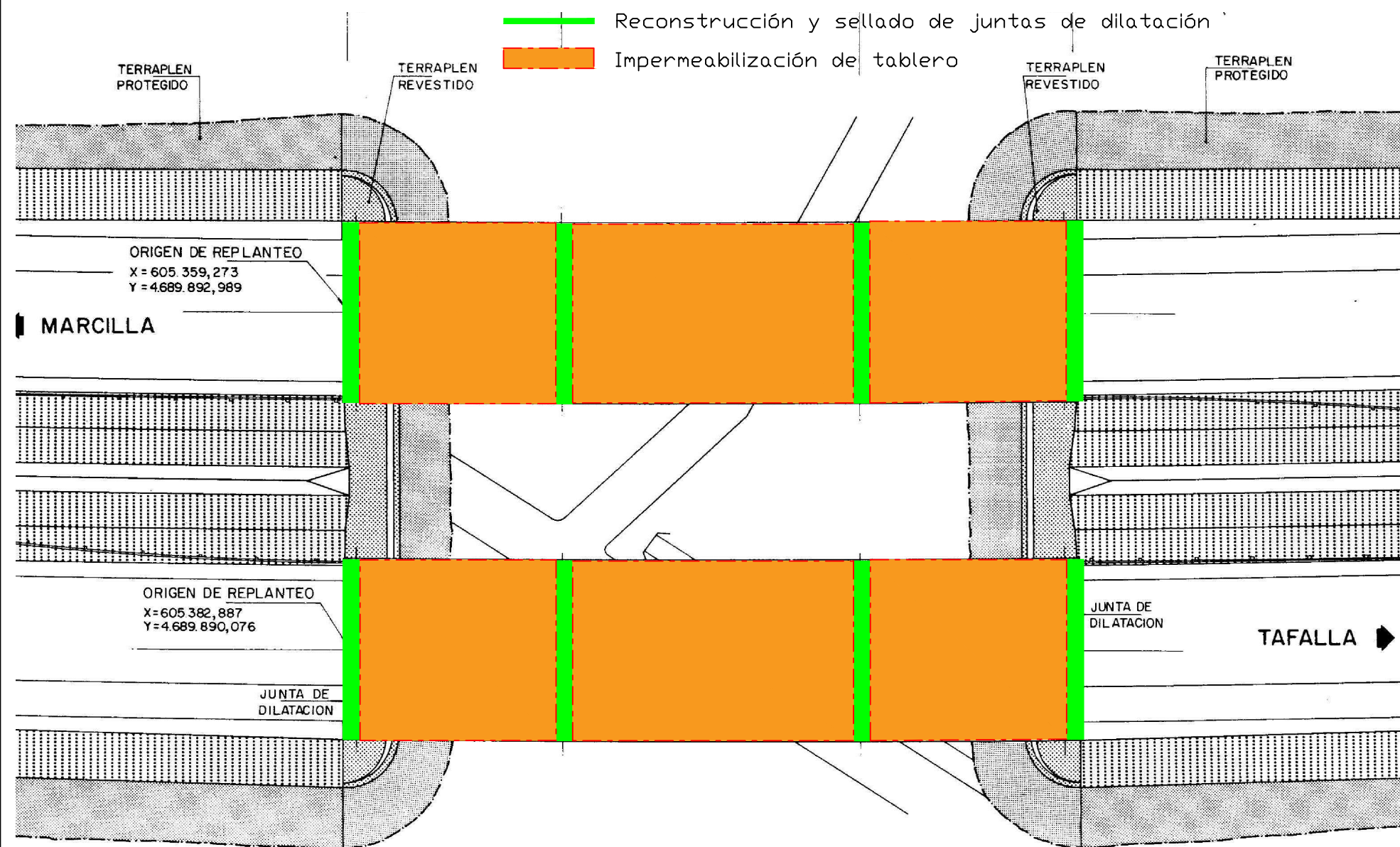
RECONSTRUCCIÓN DE ESTRUCTURAL LABIOS JUNTAS (INFERIOR)
