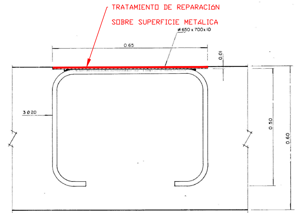
SECCION A-A ESCALA 1:5
