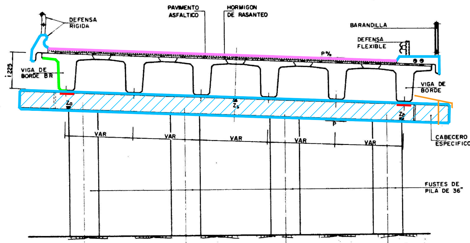
SECCION TRANSVERSAL TIPO
