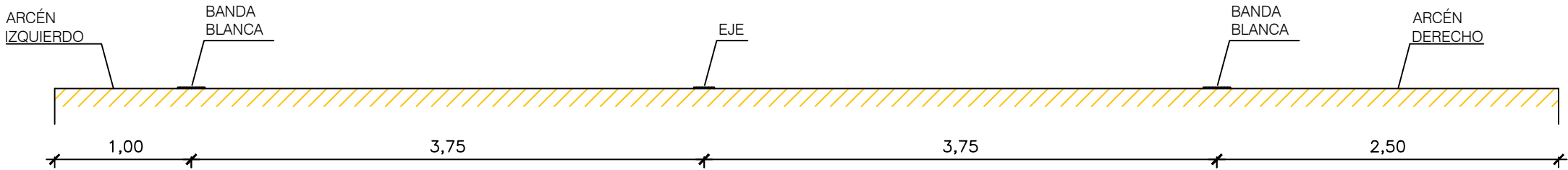
MODIFICACIÓN PROVISIONAL CALZADA A SECCIÓN EN BY-PASS
