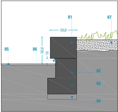
DETALLE CONSTRUCTIVO BANCO URBANIZACION
