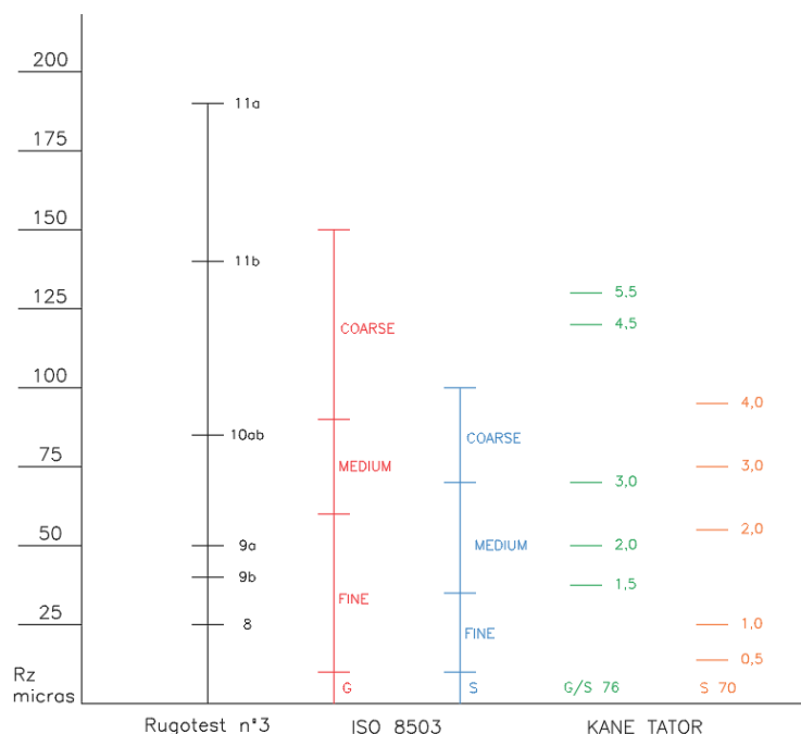
Figura 4. Relación de medidas de rugosidad según comparador.
