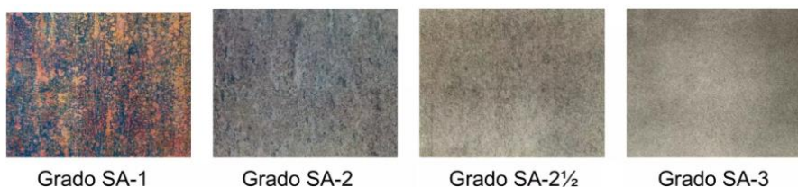
Figura 3. Patrones de limpieza para certificación visual de la superficie según ISO 8501-1.
