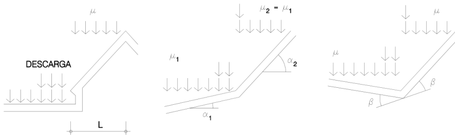
Figura 12. Coeficientes de forma en faldones según CTE-DB-SE-AE.
