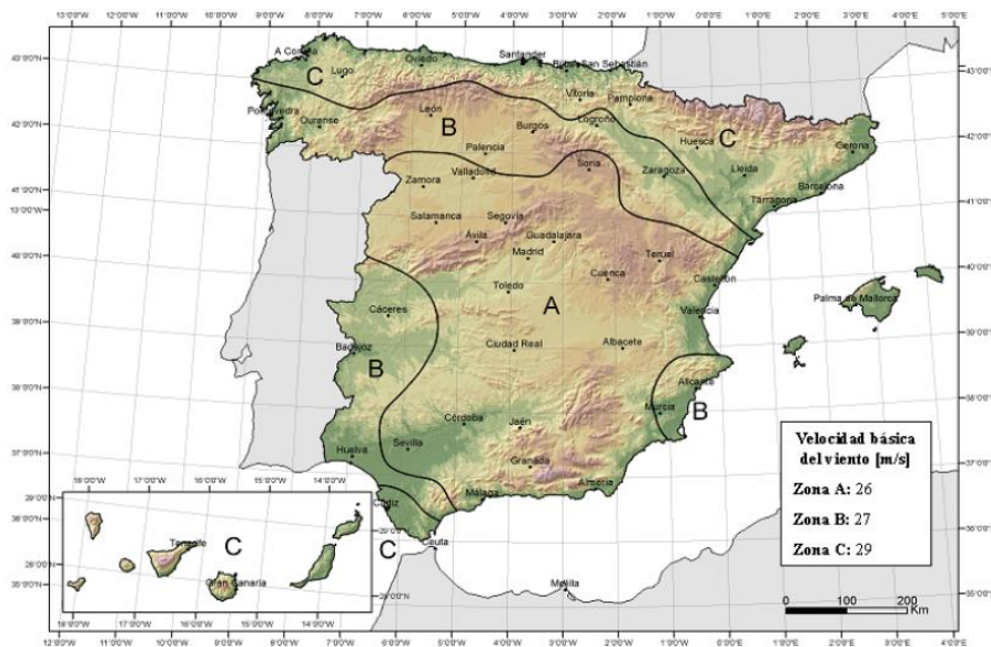
Figura 7. Velocidades básicas del viento propuestas por el CTE-DB-SE-AE.
