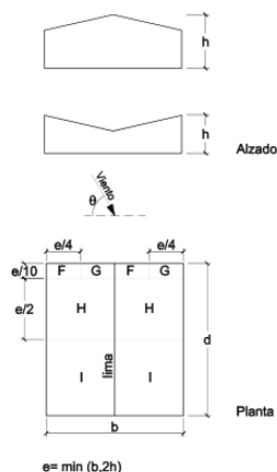
Figura 10. Coeficientes de presión sobre cubierta a dos aguas según CTE-DB-SE-AE.
