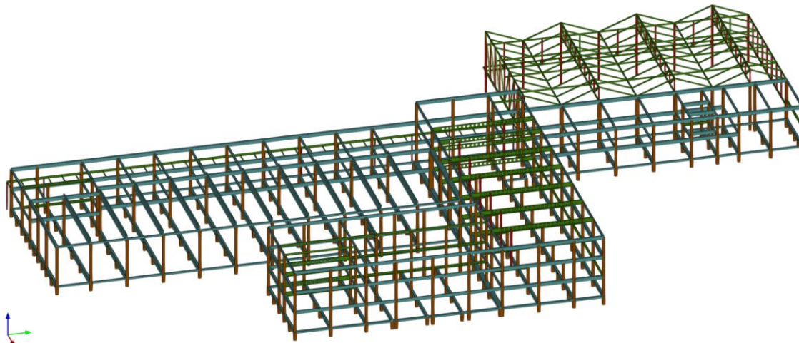
Figura 15. Modelo de cálculo global de la estructura de hormigón y cubierta metálica exterior.
