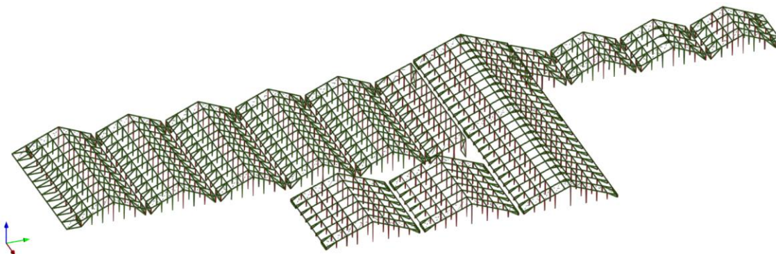
Figura 16. Modelo de cálculo global de la estructura metálica de cubierta.
