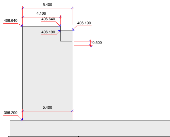
ALZADO ALETA 1
