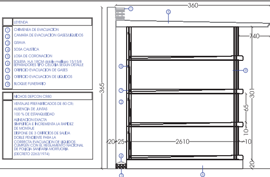
SECCIÓN CONSTRUCTIVA
