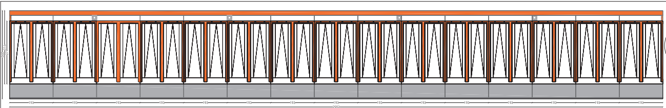
PLANTA DE LOS NICHOS
