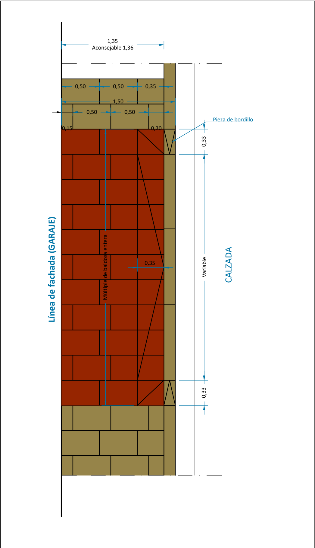
Detalle replanteo "Acceso vados" s:1/30
