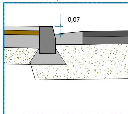
Detalle altura bordillo s:1/20
