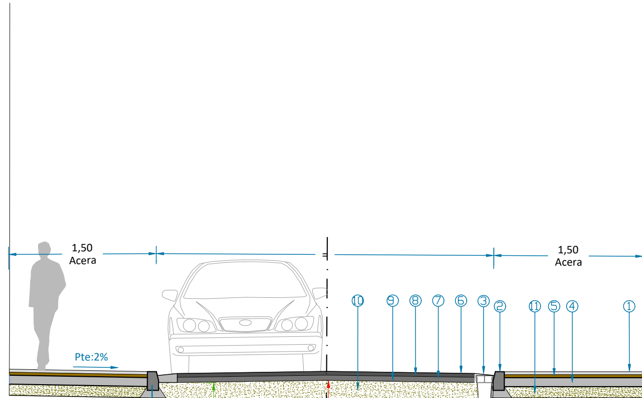
SECCIÓN TIPO CALLE s:1/50
