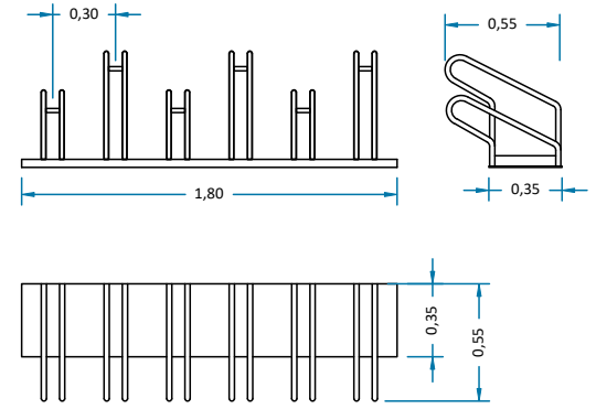
Detalle aparcamiento bicicletas s:1/25
