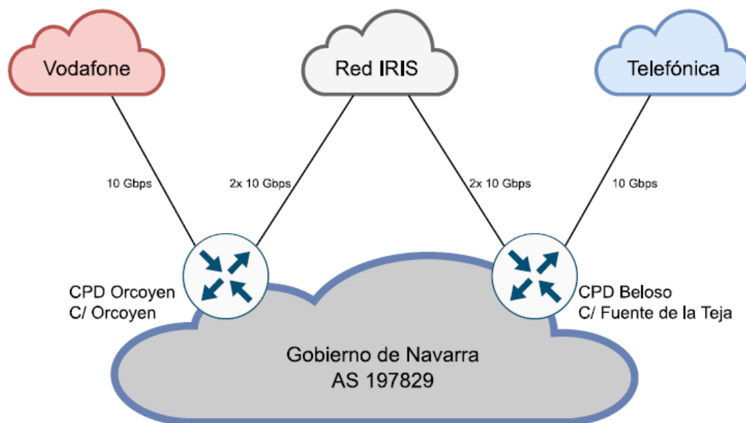
Figura 1: Esquema actual de tránsitos a Internet de GN
