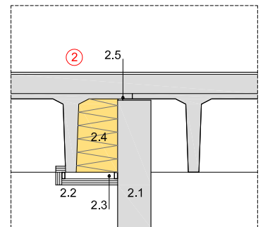
DETALLE SELLADO GRIETA SUPERIOR
