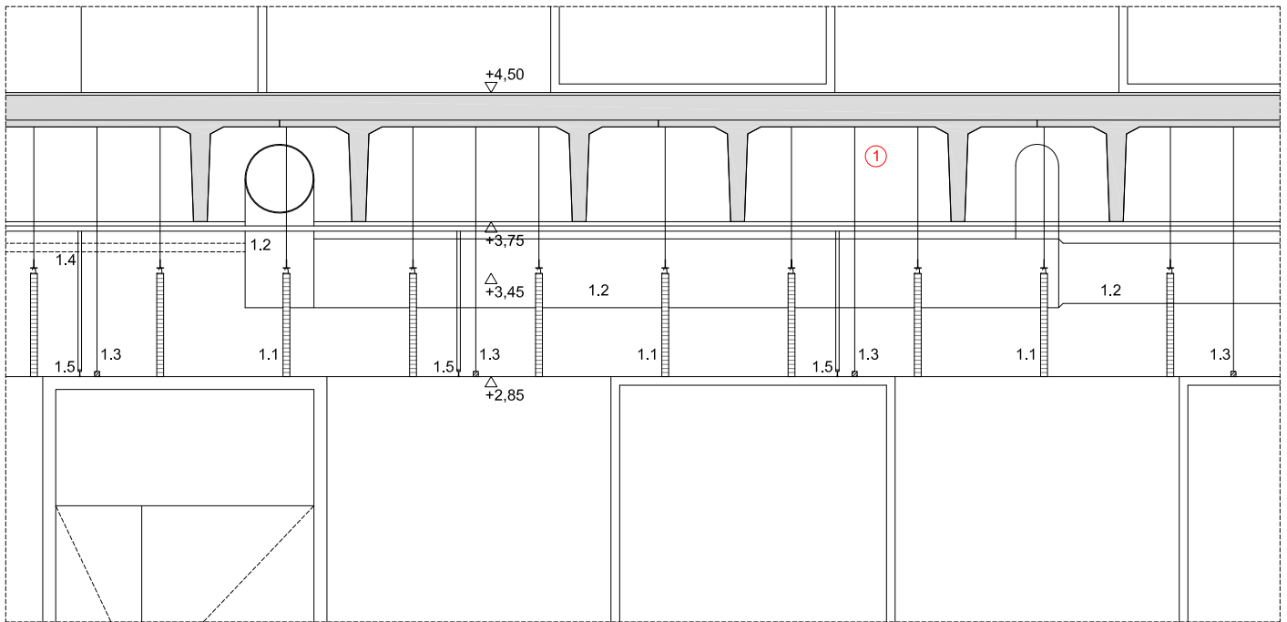
DETALLE SECCIÓN LONGITUDINAL
