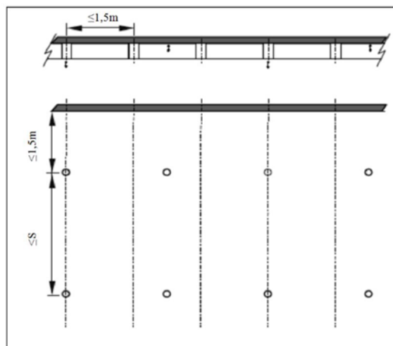
Disposición de rociadores bajo techos con vigas formando canales, vista en alzado (arriba) y en planta (abajo)
