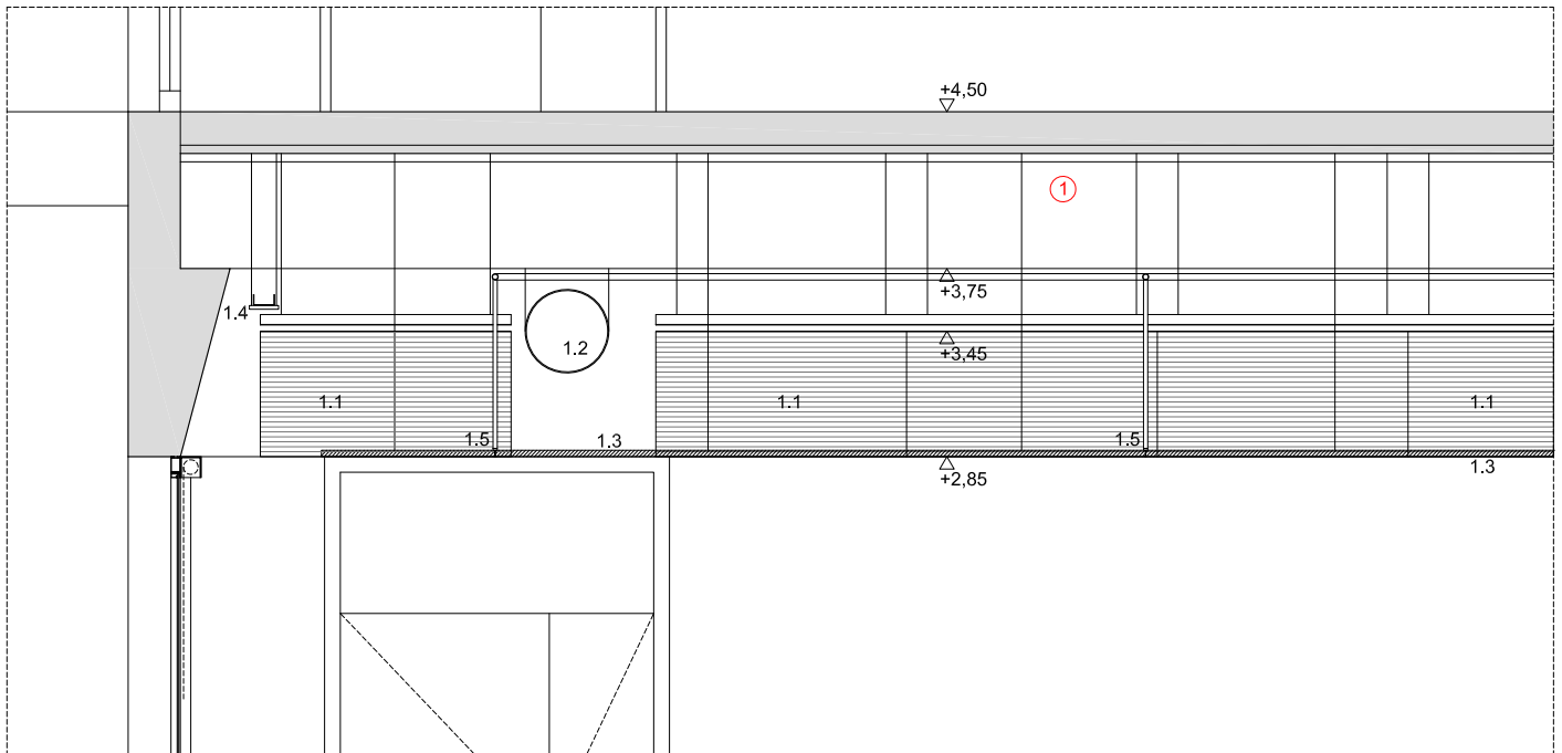
DETALLE SECCIÓN TRANSVERSAL
