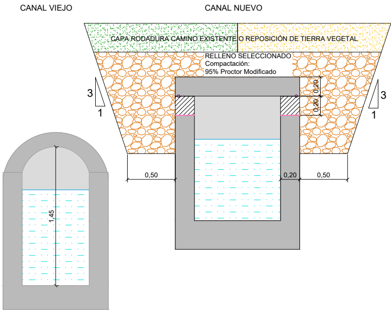
SECCIÓN RELLENO REPOSICIÓN LOSA EXISTENTE POR NUEVA LOSA
