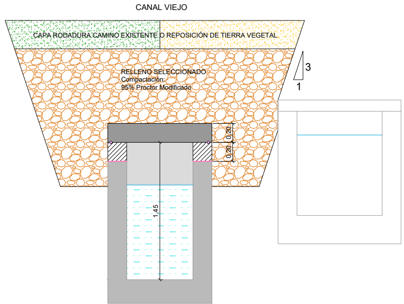
SECCIÓN RELLENO REPOSICIÓN DE BÓVEDA POR LOSA
