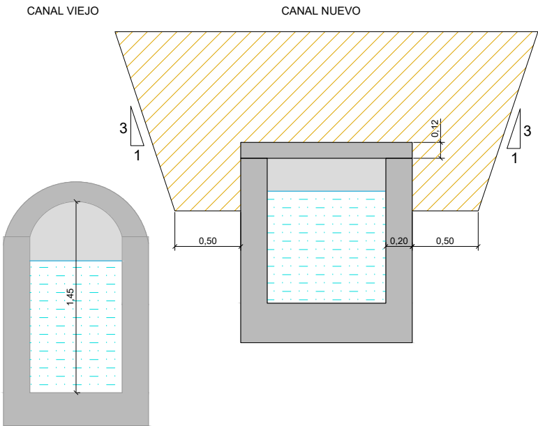
SECCIÓN DEMOLICIÓN Y EXCAVACIÓN REPOSICIÓN LOSA EXISTENTE POR NUEVA LOSA
