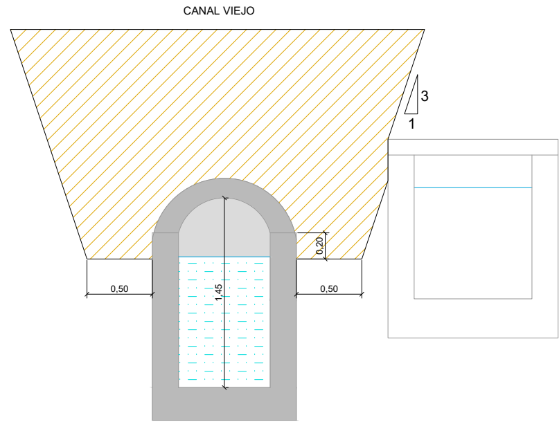
SECCIÓN DEMOLICIÓN Y EXCAVACIÓN REPOSICIÓN BÓVEDA POR LOSA
