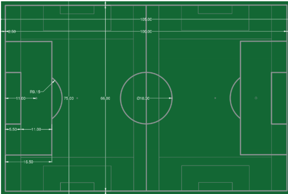
Dimensiones del campo de fútbol 11 según normativa NIDE.
