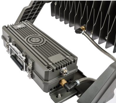
Driver instalado en la parte posterior del proyector, en una caja IP66.
