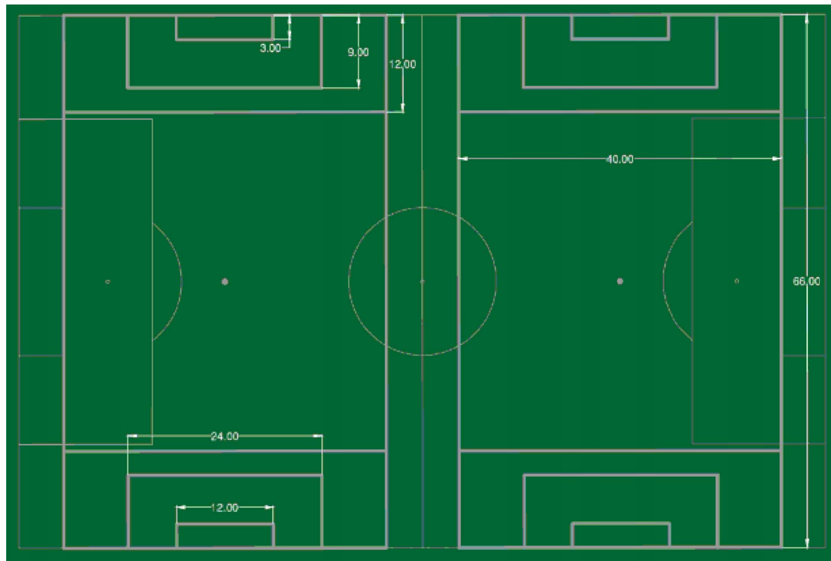
CAMPO DE FÚTBOL 7
