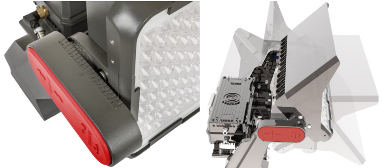
El proyector se puede regular hasta 270°
