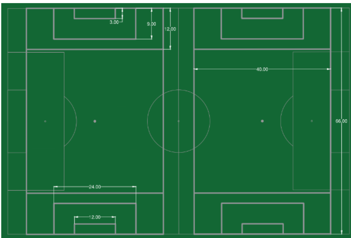
Dimensiones del campo de fútbol 7 (dos unidades) según normativa NIDE.
