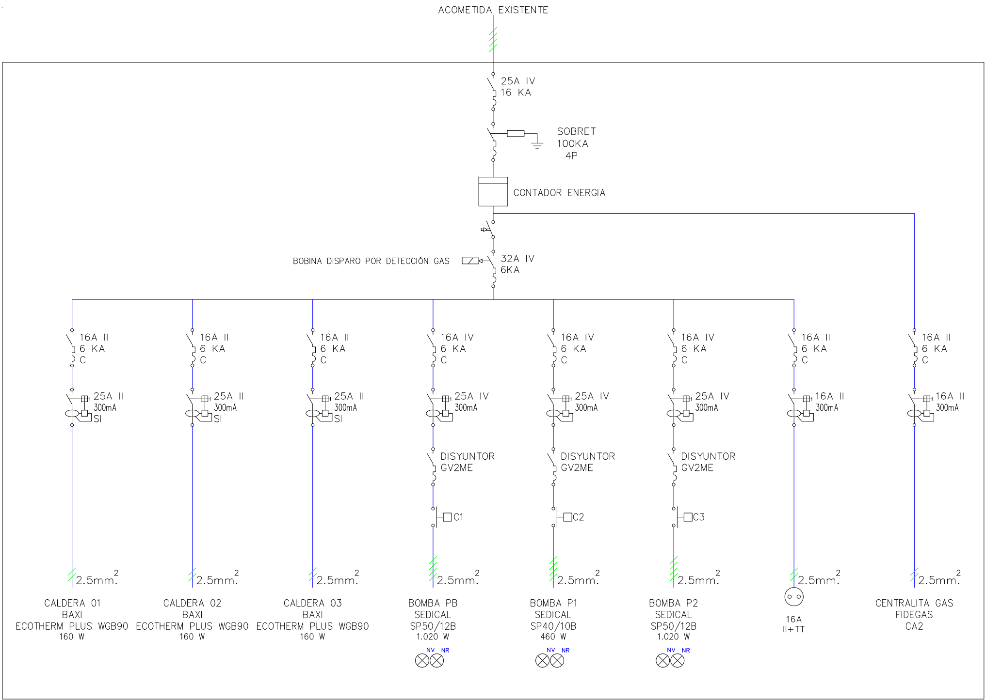
CUADRO INSTALACIÓN DE CALEFACCIÓN
